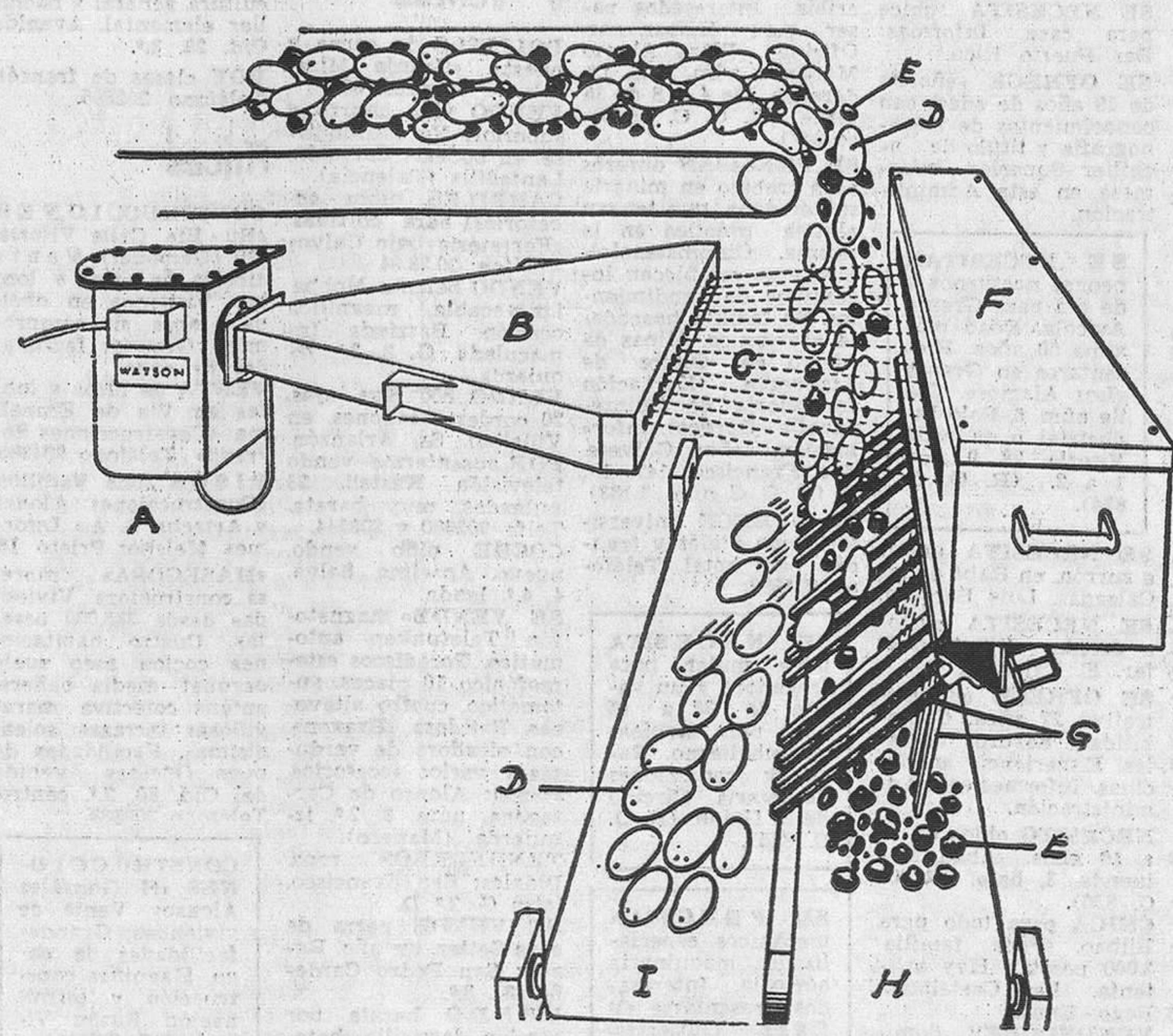
Diseño de una máquina limpiadora de patatas
