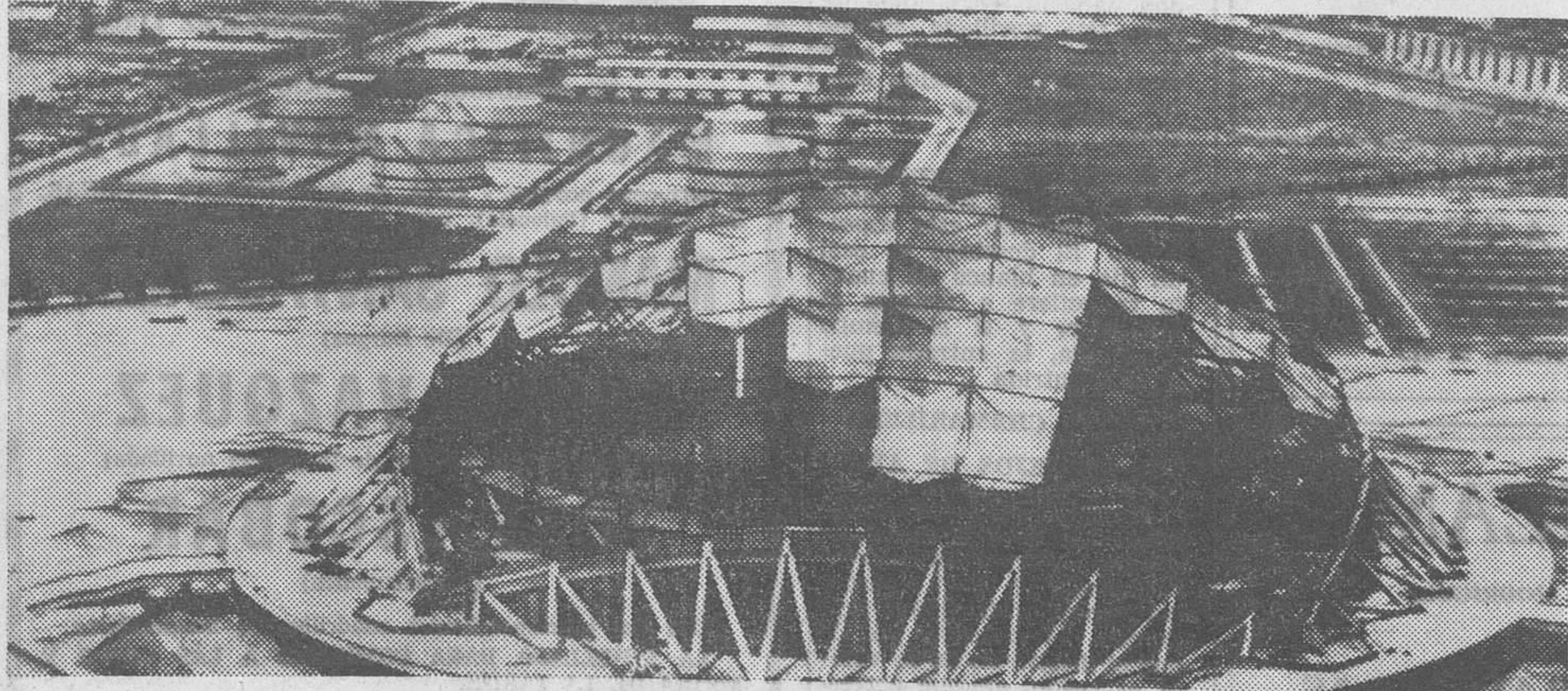
Méjico. — El Palacio de los Deportes de Mixhuca, cuya construcción estará lista para los Juegos Olímpicos con capacidad para unos 22.000 espectadores, podrán celebrarse en él pruebas de atletismo en pista cubierta, balón-volea, hockey sobre hielo y baloncesto. — (Telefoto UPI-CIFRA)
