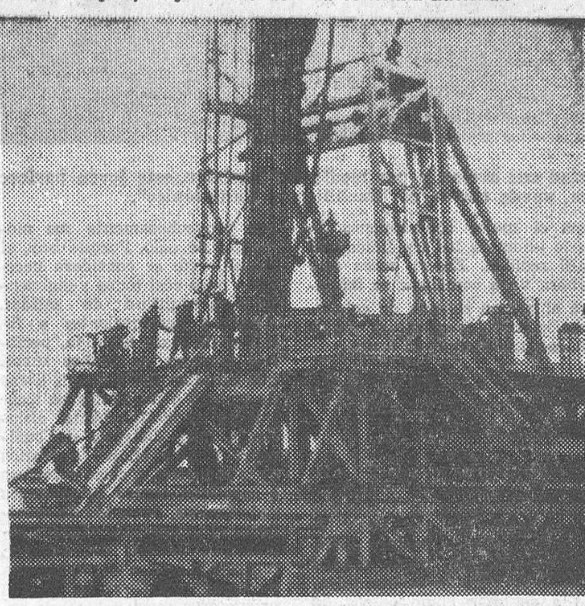
El personal del tren de sondeo del «Ayoluengo número 2» en plena acción de su trabajo, durante las maniobras con el largo varillaje de acero.—(Foto FEDE)
