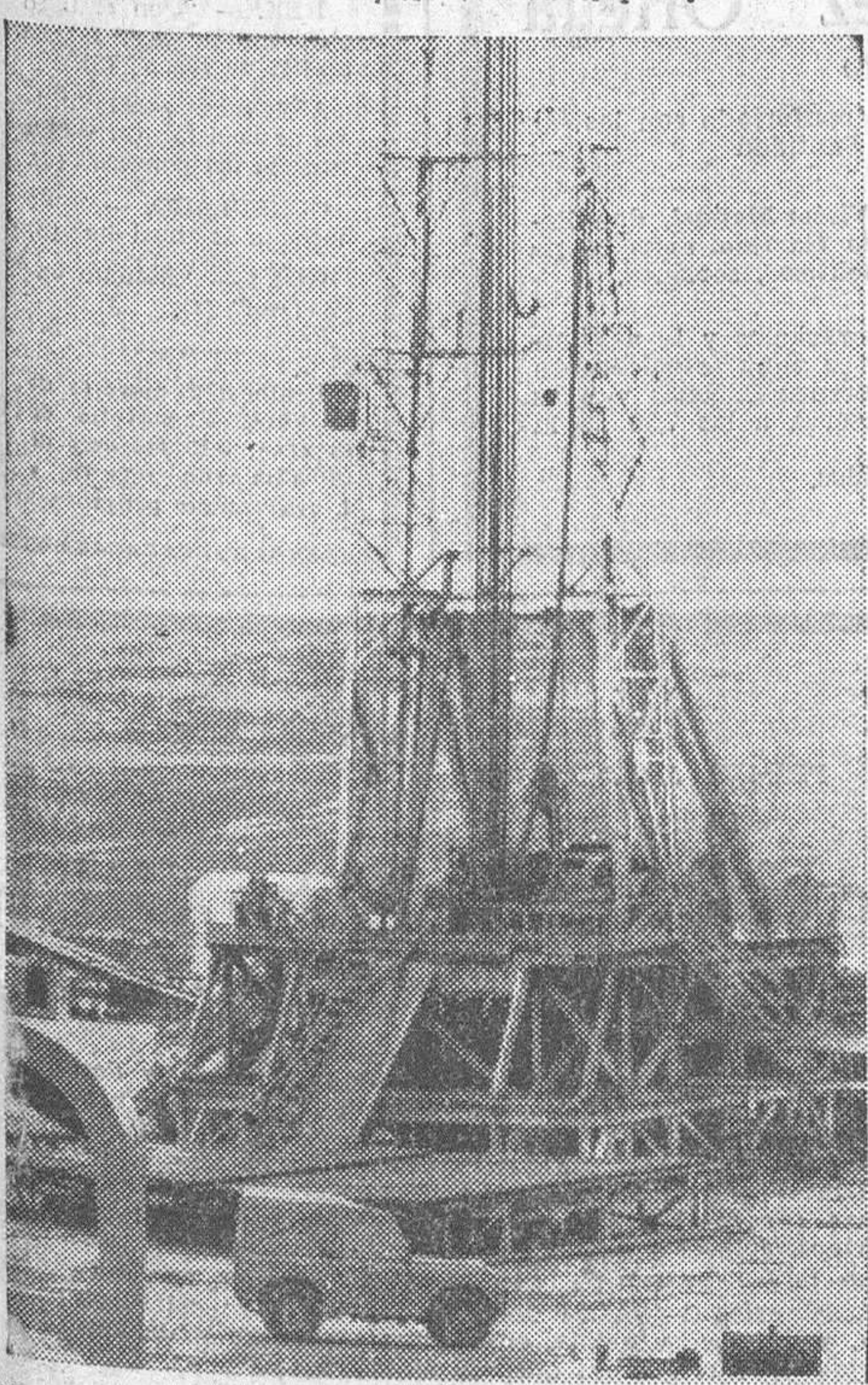
Estas imágenes fueron ayer captadas por "Fede" en el páramo de La Lora. En el grabado de la izquierda se reproduce un aspecto del tren de sondas en el «Ayoluengo número 2», mientras que la panorámica muestra una perspectiva general del tercer campamento petrolífero. La "foto" recoge el instante en que es izado el castillete del nuevo tren de perforación.
