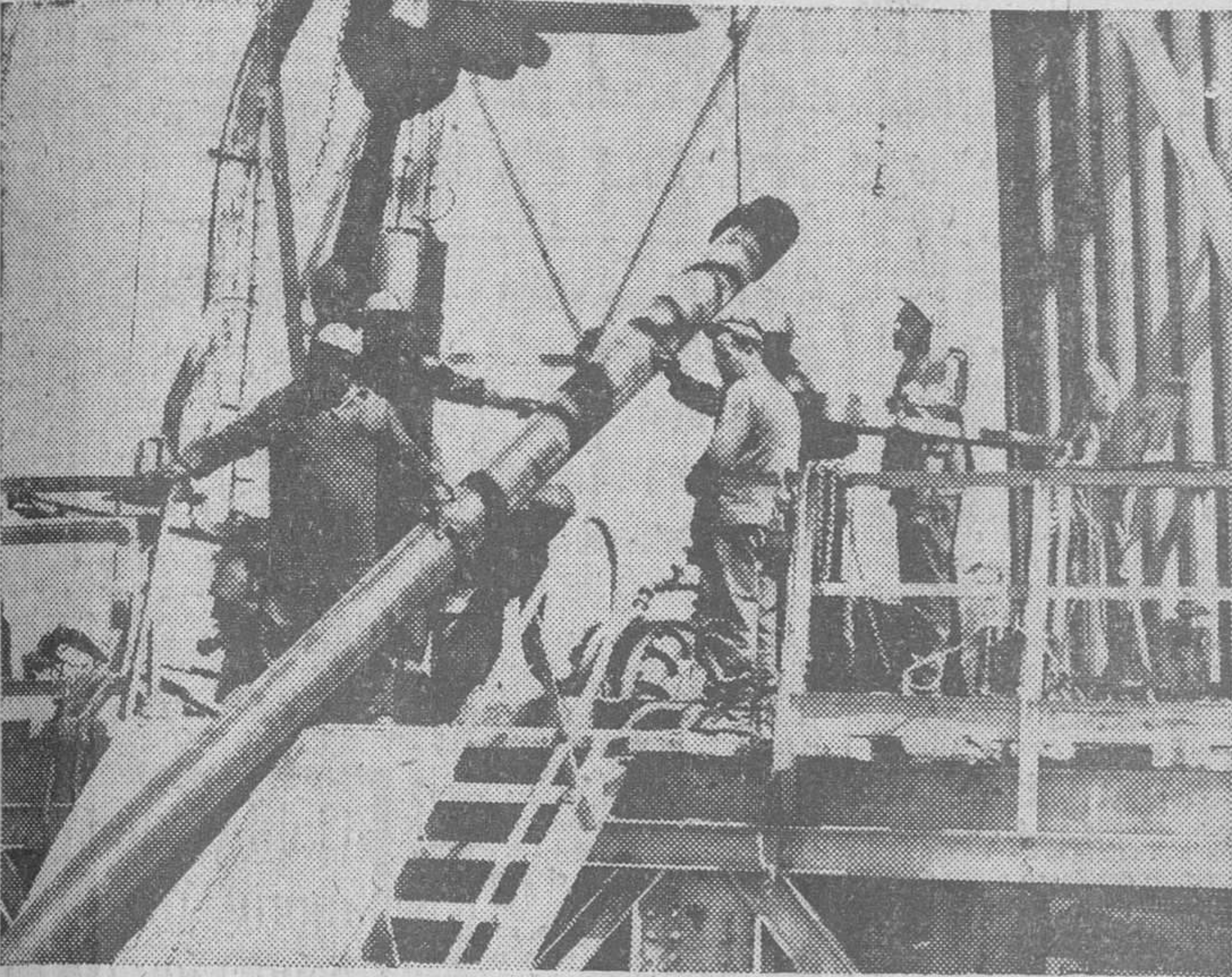
Este es el momento en que en la torre de perforación de Valdeajos, es izado uno de los tubos de acero, durante la fase de los trabajos de entubado que consiste en introducir en el pozo hasta la profundidad de 1.500 metros que alcanza el actual sondeo, todo el sistema de tuberías, antes de procederse a la cimentación de las paredes del hueco. (Foto FEDE)
