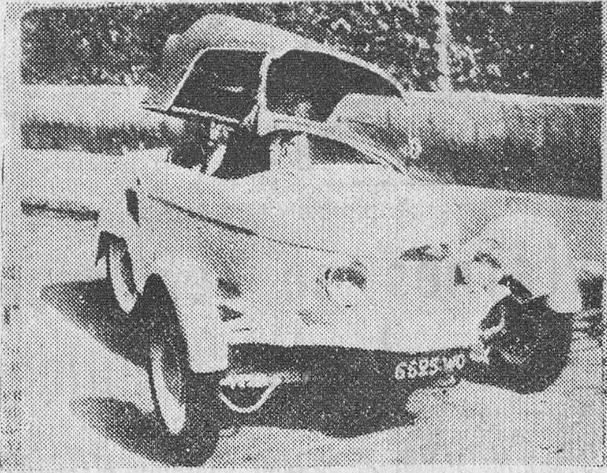
Un artesano francés Mr. Robert Hannoyer, va a presentar en el Salón del Automóvil un pequeño vehículo de un caballo de fuerza, cuya velocidad es de 80 kilómetros hora, con un consumo de tres litros y medio de gasolina cada cien kilómetros. Posee además una carrocería desmontable y plegable, lo que permite poder guardar el vehículo en un espacio reducido. (Foto Gil del Espinar)
