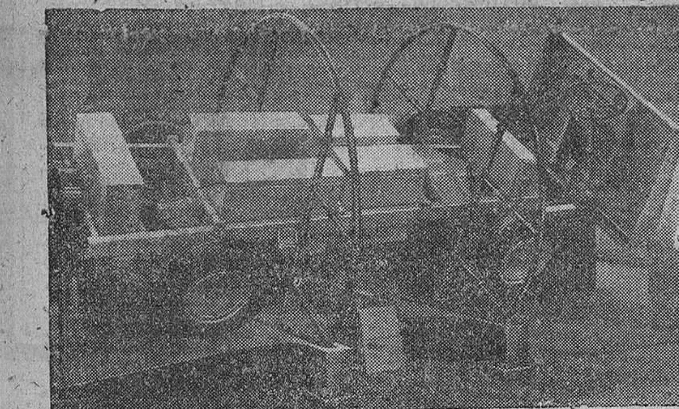
Este nuevo chasis que se ha exhibido en una exposición recientemente celebrada en Londres, es de gran utilidad para las empresas que tienen que hacer repartos casa por casa, como lecherías, panaderías, etc. Está accionado por una batería con control de retraso automático y descarga automáticamente la mercancía por un sistema de mandos montado en la cabina.—Foto CALPE.
