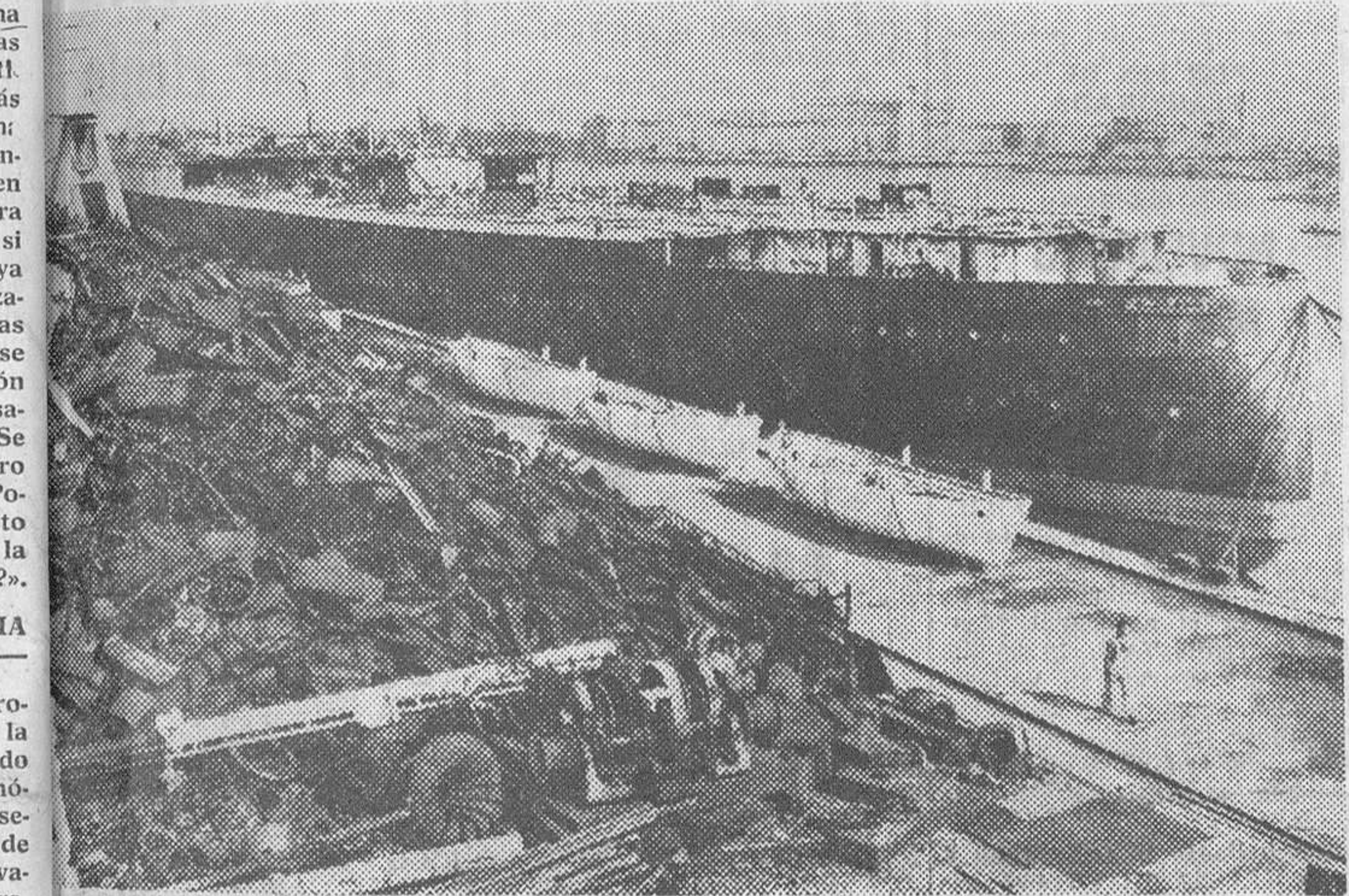
El «Hanseatic», buque alemán de 30.000 toneladas está siendo convertido en chatarra en el astillero de buques de Waltersjöf, en Hamburgo. En la fotografía vemos el gran montón de chatarra que ya se ha sacado de él. Sólo queda por desmontar el casco. — (Foto FIEL).
