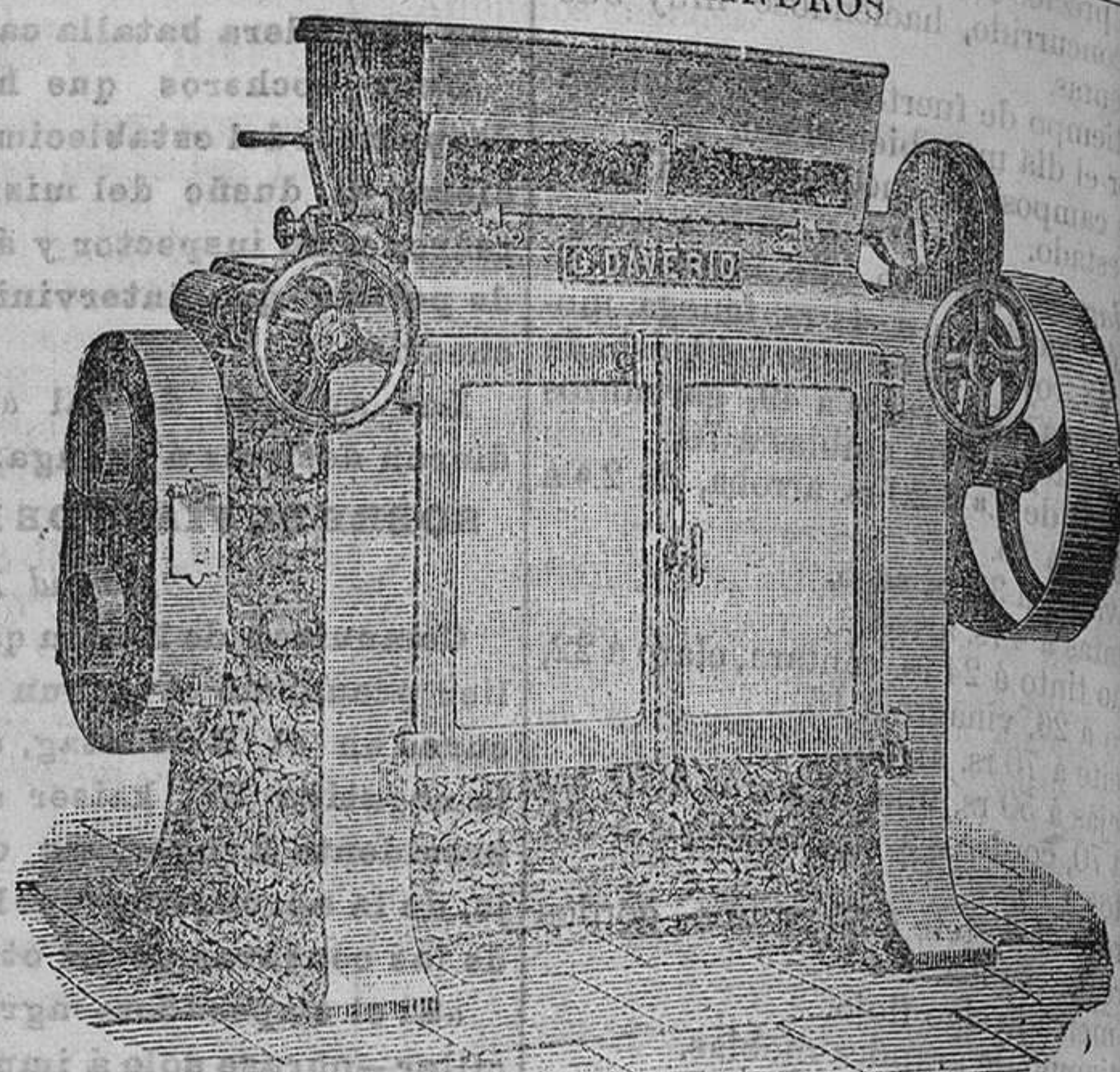
PLANSICHTER (último modelo).— Construcción Daverio.
