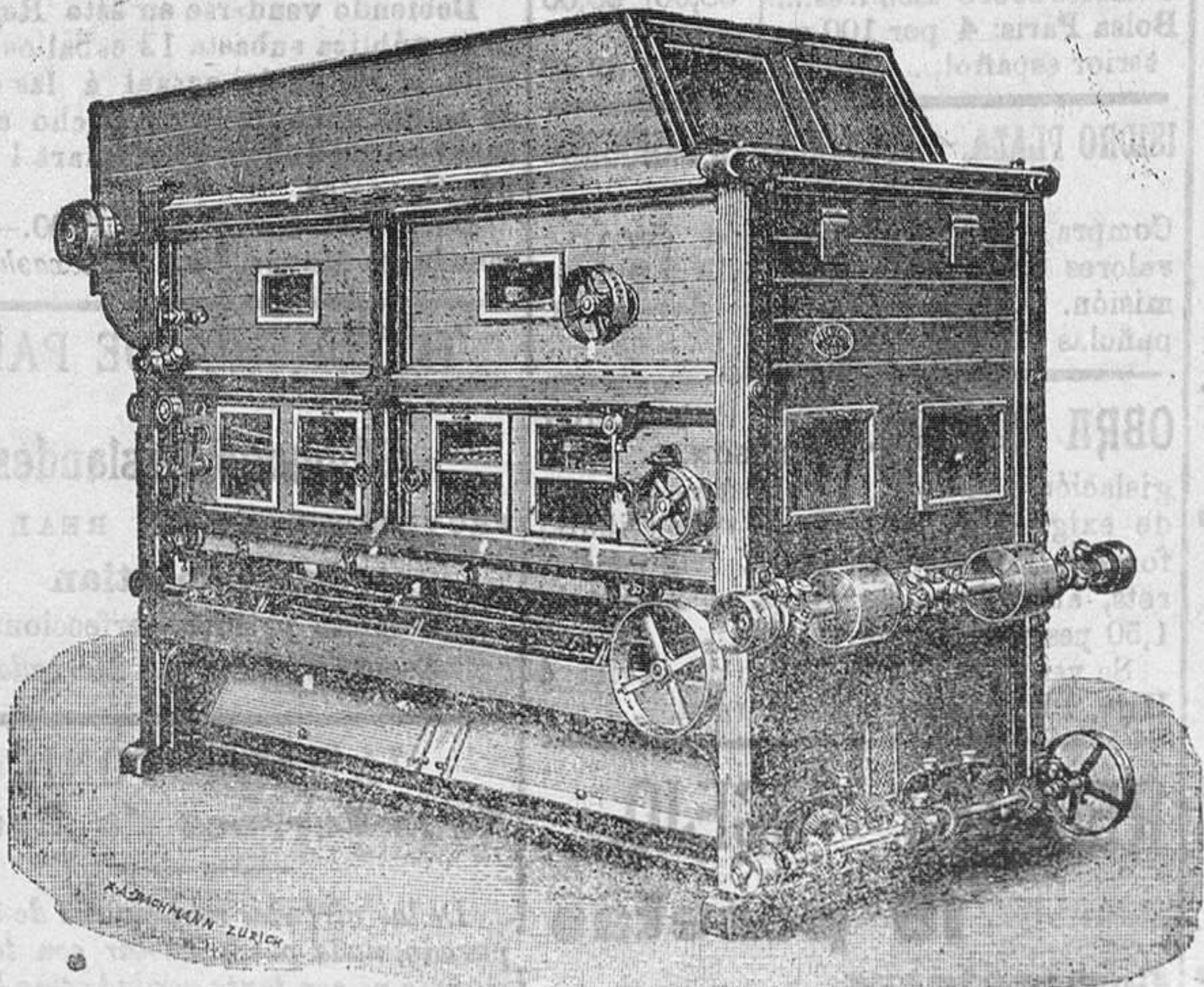
COLUMNA DESPUNTADORA
