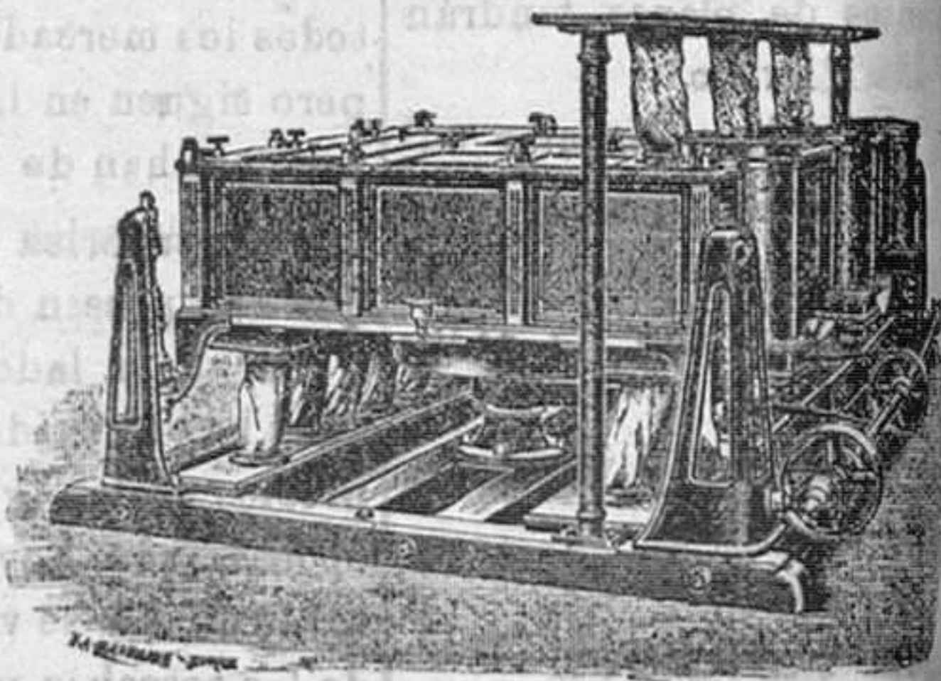
PLANSICHTER (último modelo).--Construcción
