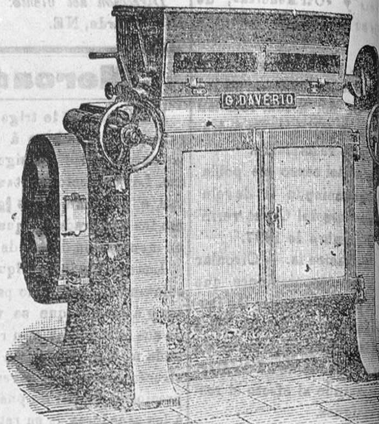
PLANSICHTER (último modelo).--Construcción
