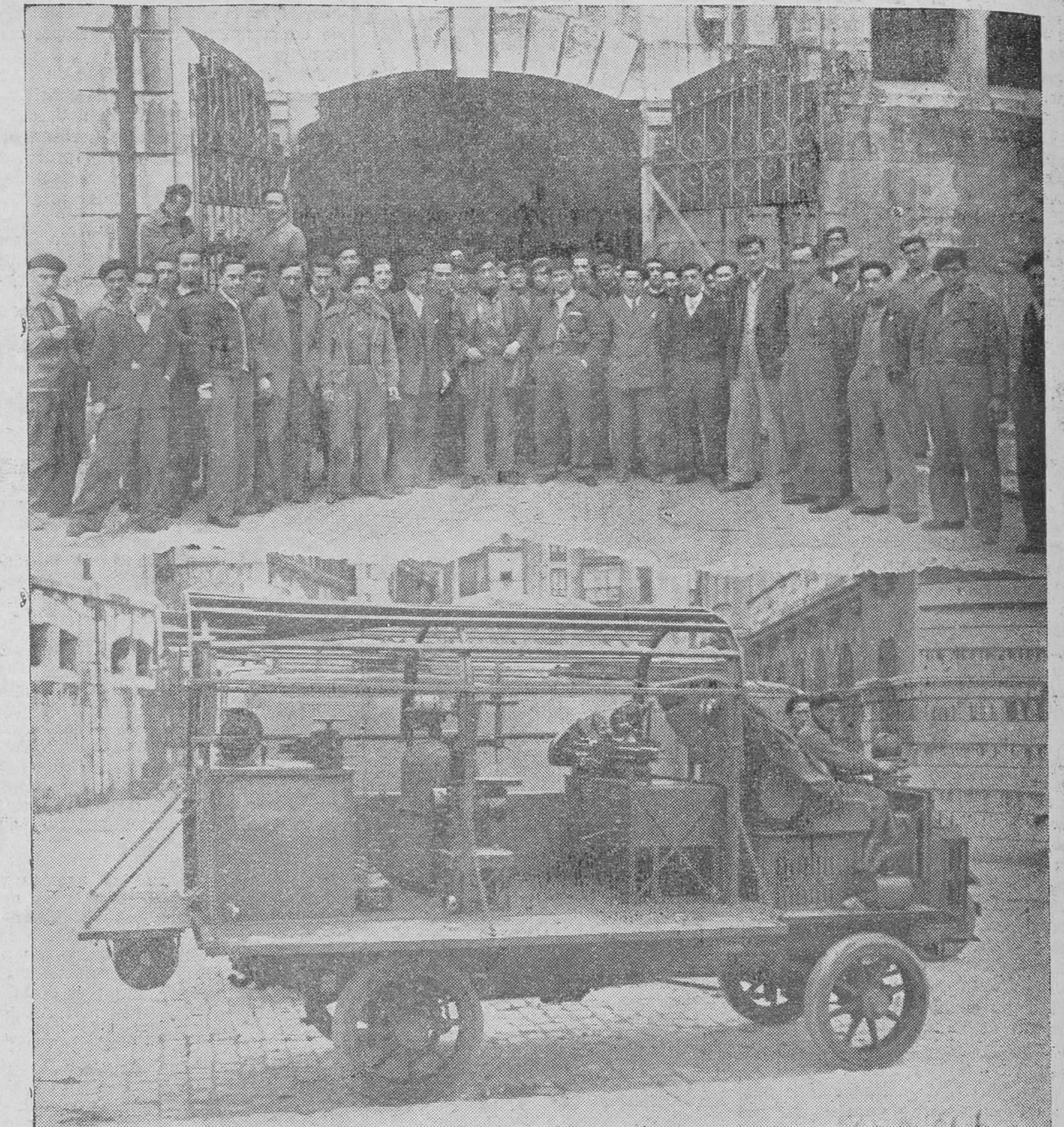
El servicio de transportes de gasolina funciona con gran regularidad gracias al acierto y trabajos de los componentes del Parque Móvil. En la foto, «Samot» ha recogido un interesante y práctico taller mecánico sobre ruedas y un grupo de jefes y personal del Parque y Talleres.
