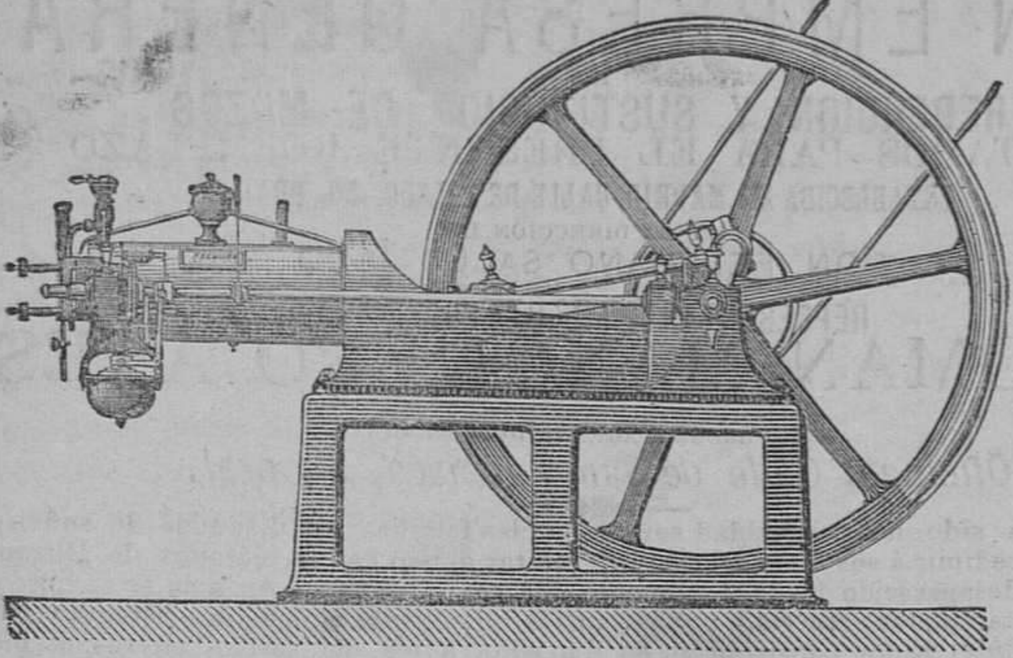
se quiera, con sólo dos ó tres días de trabajo.—Los motores de ESCUDER, no llegan á consumir un metro cúbico de gas por hora y po caballo, no teniendo necesidad de ningún empleado para cuidarlos...
