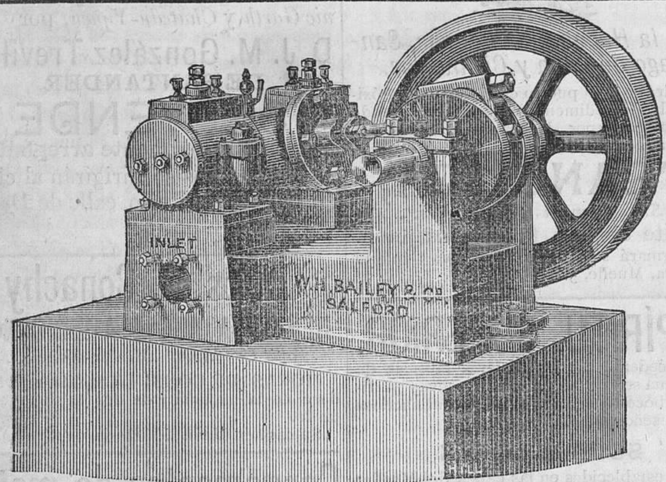
MOTORES HIDRAULICOS.
