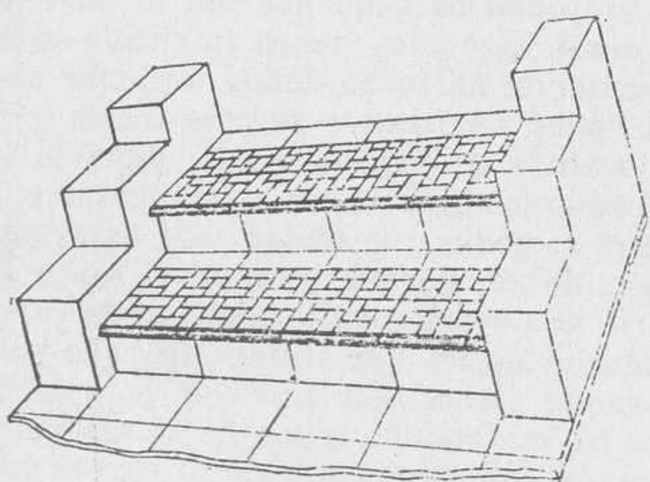
Escalera con pasos antirresbalable "CRESPO"
