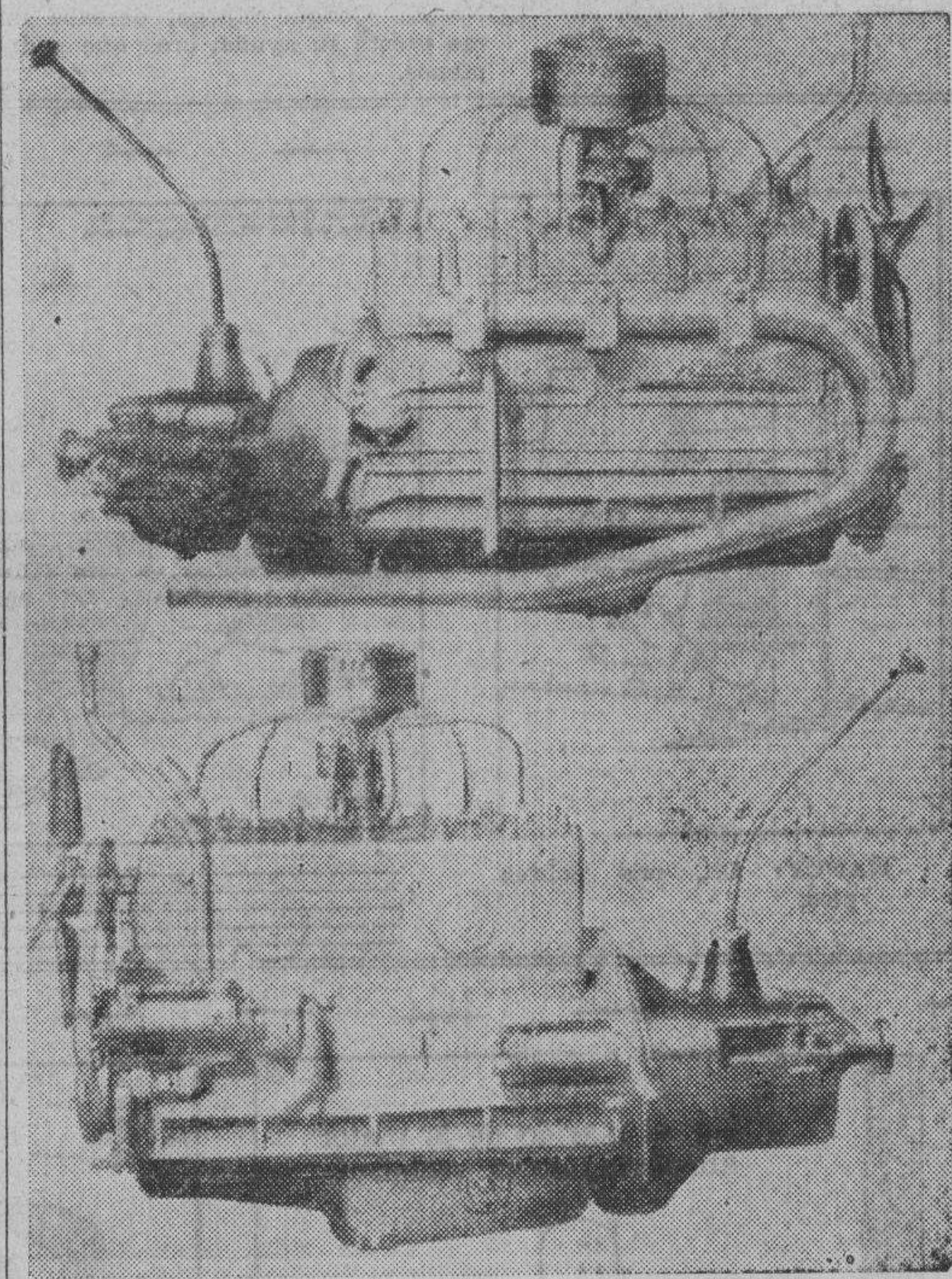
Nótese en el cliché que publicamos la parte derecha del motor del nuevo Nash "400" que ahora se vende en Filipinas, del tipo de motor sellado. Abajo aparece otra reproducción del mismo motor visto desde otro ángulo. En las dos figuras el lector notará que no existe ninguna parte que se encuentre fuera del bloque. Esto quiere decir que todas las partes de este motor funcionan dentro, sin la intervención del hombre y con la simplicidad y seguridad nunca vistas en ningún motor fabricado hace diez años.
