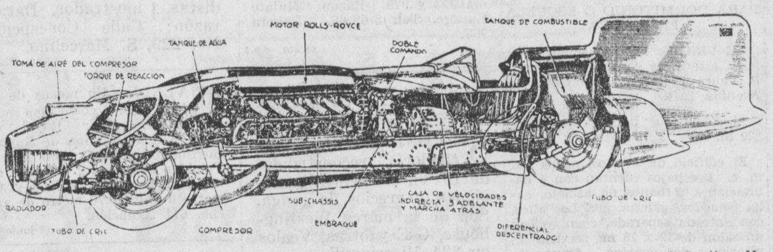
Una demostración de los principales organos de "Blue Bird" reformado, con el que el Capitán Malcolm Campbell mejoró últimamente su propio record de velocidad llegando, en el kilometro lanzado, ida y regreso, a un promedio de 480 kilometros por hora, o sean 272,463 millas por hora. El motor es un Rolls Royce de 12 cilindros, sobrealimentado, con una fuerza de 2,500 caballos de vapor, siendo el peso total del coche, en orden de marcha, 4,500 kilogramos.
