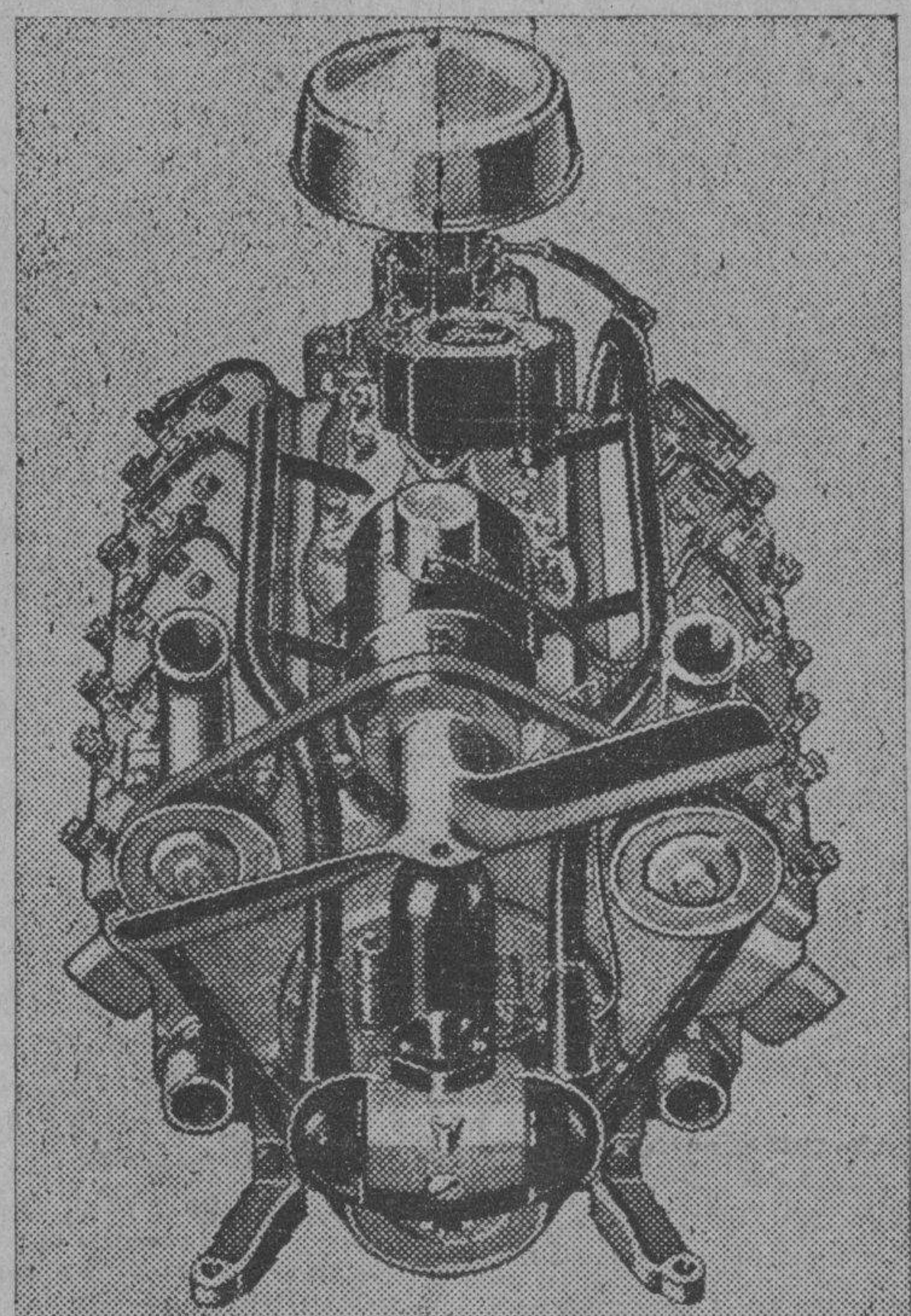
La Maquina del Nuevo Ford V-8
