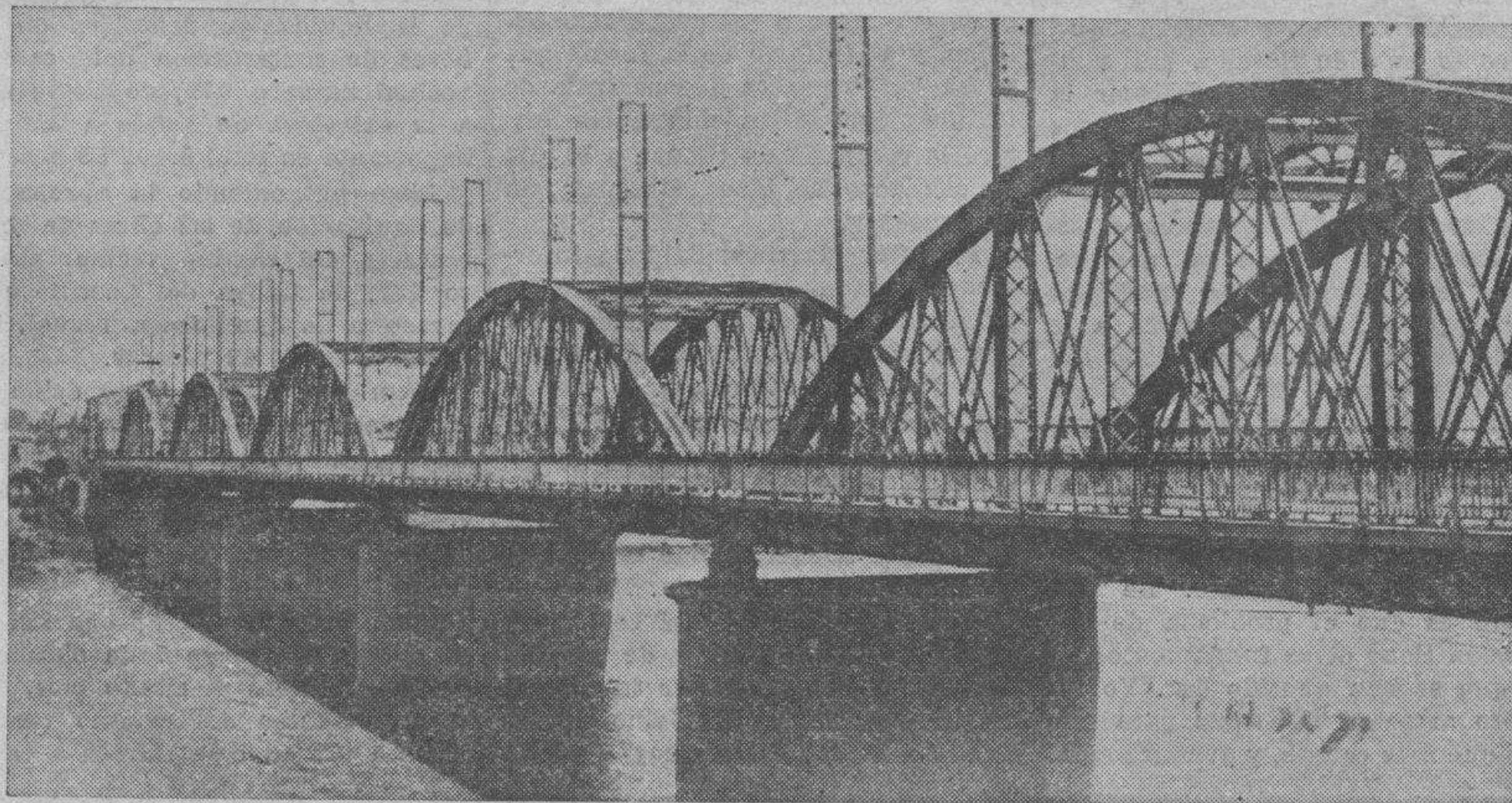
Extraño aspecto del Puente del Pilar al haberse modificado la instalación de conducciones eléctricas que había en él para servicio de la población, en la margen derecha del Ebro.
