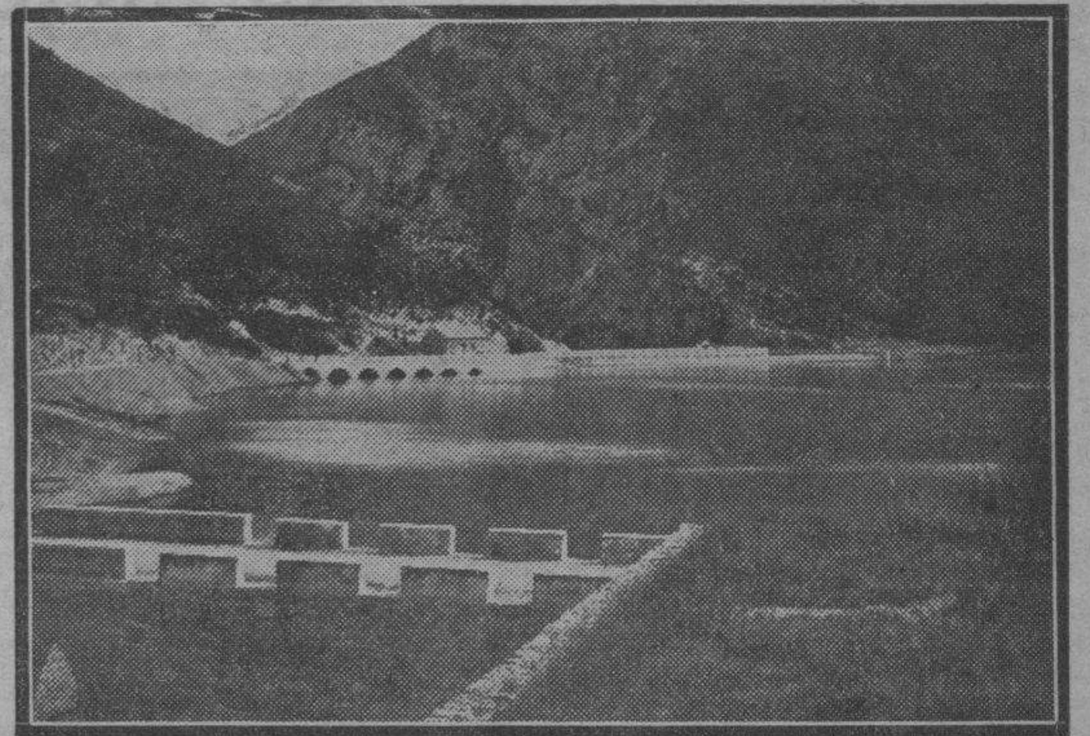
HUESCA. — La famosa presa recrecida del pantano de Arguis, verdadera nodriza de la huerta oscense. (Foto. Oltra)
