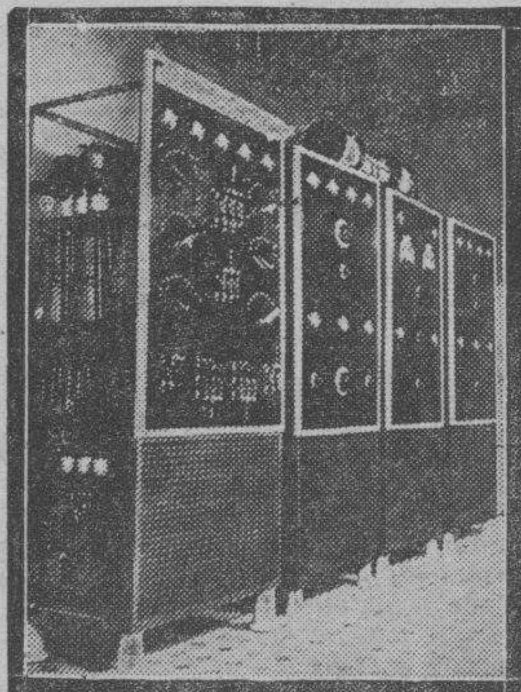
Conjunto completo de una emisora terminada.
