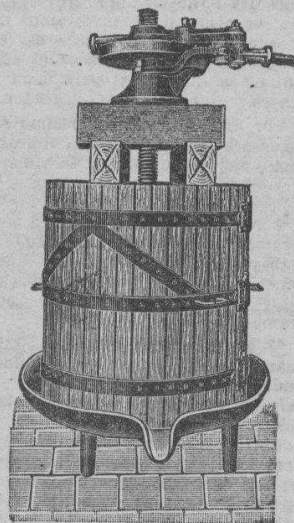
Prensa para vino, de especial construcción, de AVERLY, S. A.
