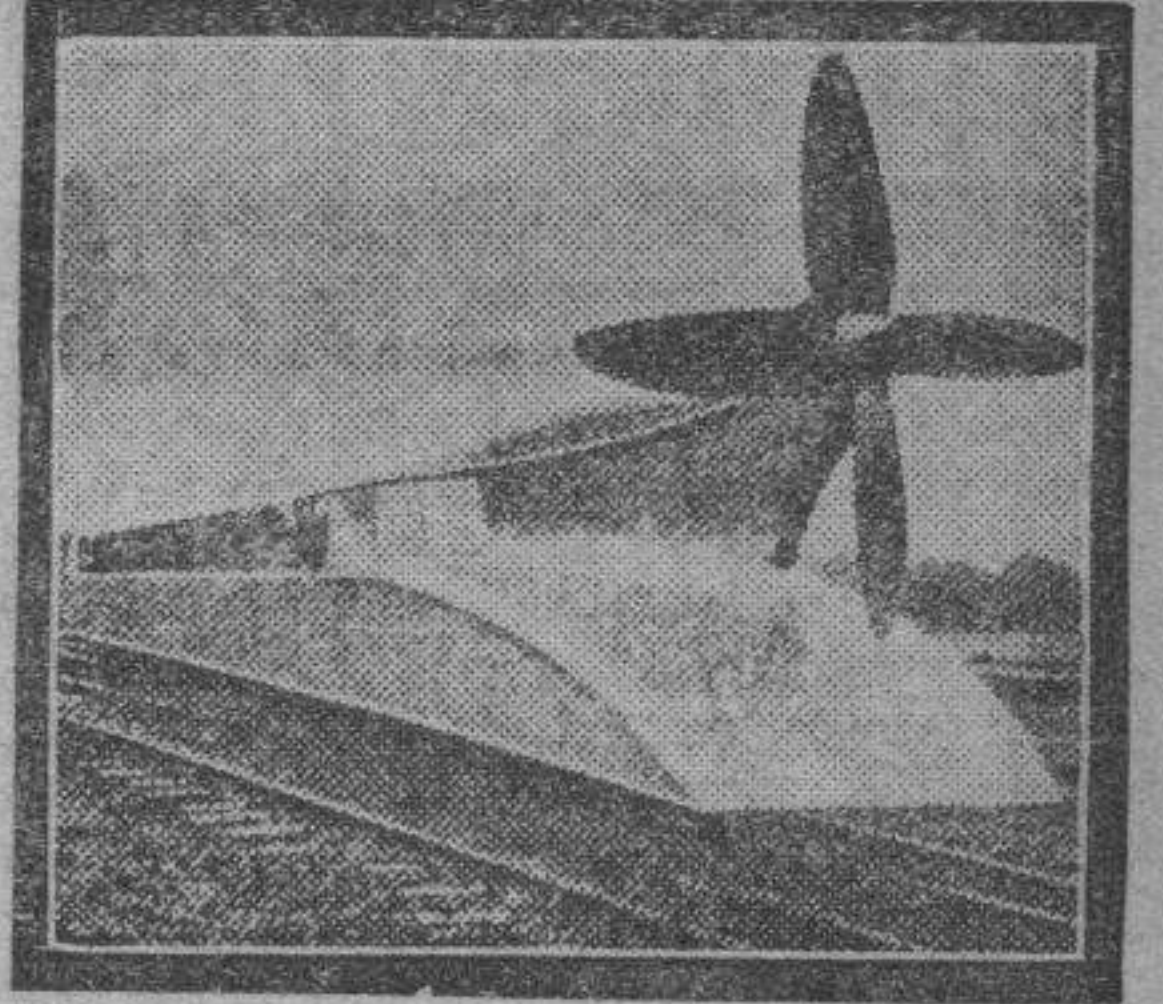
Parte posterior del tren a hélice y cabina de los motores. El moderno sistema de tracción proporciona al convoy unos movimientos muy suaves, y no precisa añadir peso muerto al vehículo para asegurar el rozamiento.
