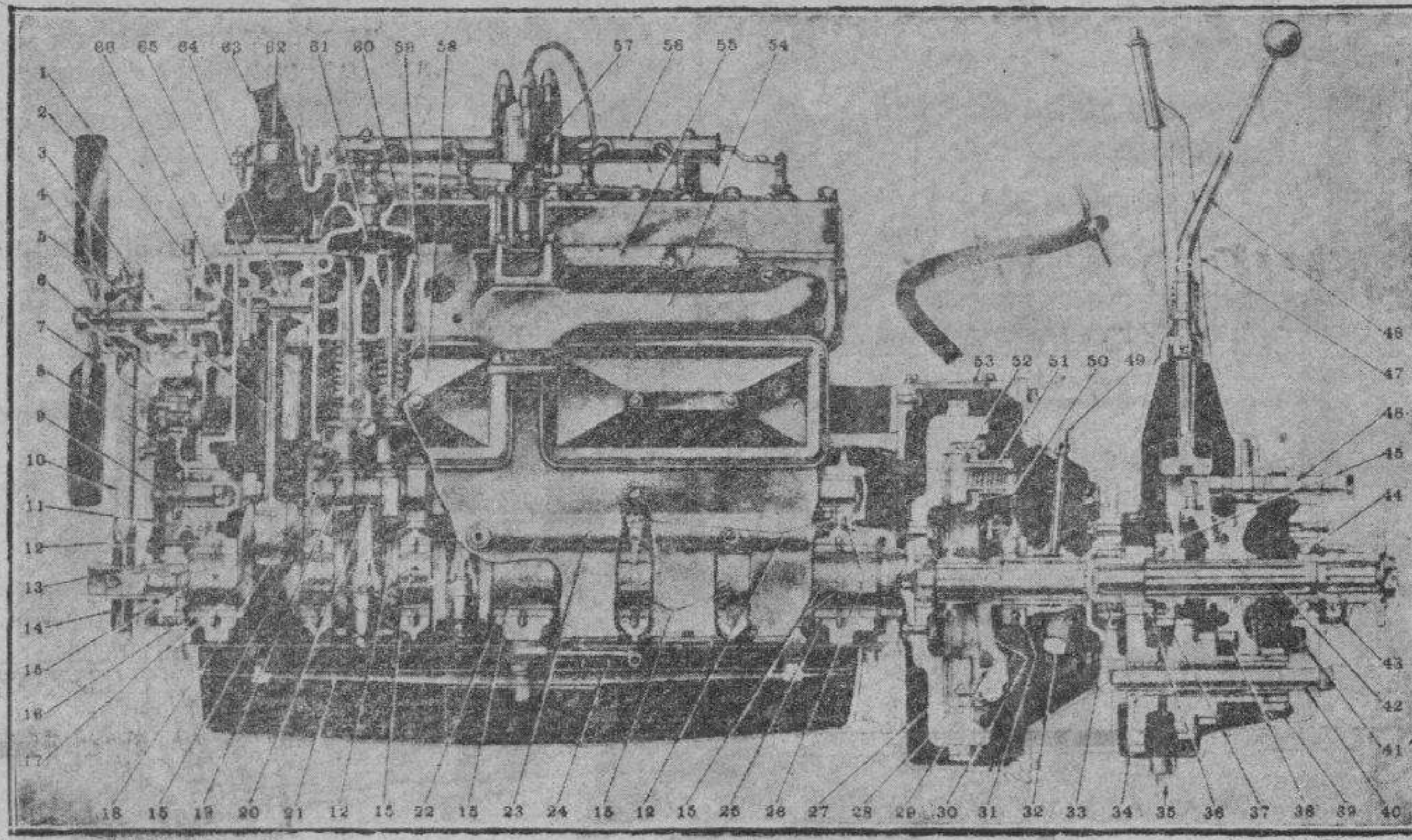
Sección del motor de la camioneta POPULAR Whippet
