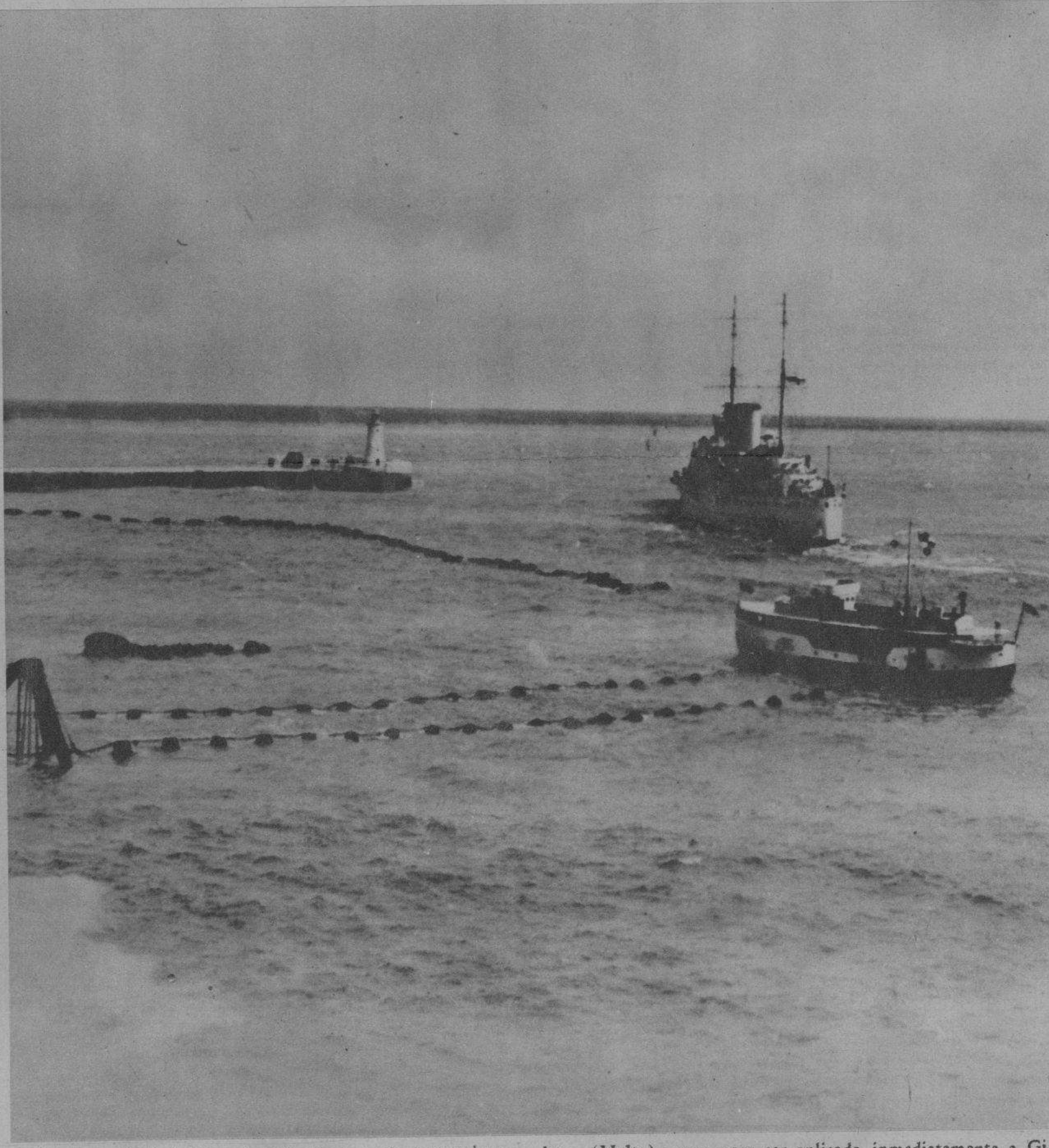
POR SU PARTE, la Gran Bretaña ha tomado precauciones en sus bases del Mediterráneo. Hace pocos días, en la isla de Malta, se ensayó este método de obstruir la entrada del puerto con unas bombas contra submarinos, a fin de cerrarlo cuando lo estimen conveniente. El ensayo hizo en la Va-
