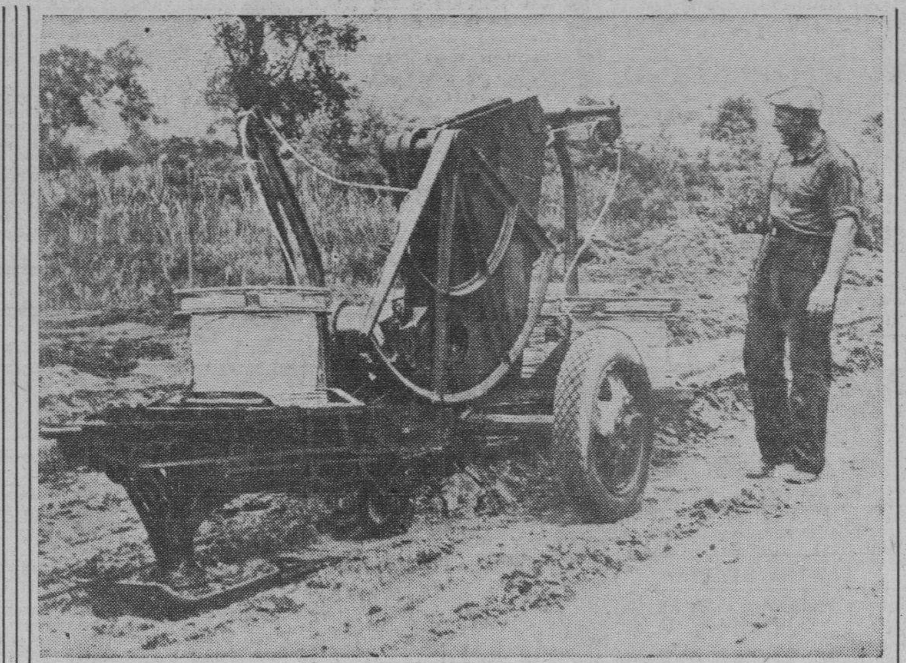
Este ingenioso aparato va perforando la tierra hasta una hondura de dos pies, según avanza, y colocando un cable telefónico, a la manera que se hace con los cables submarinos. Lo que no sabemos es lo que pasará si encuentra una roca viva. Lugar de la invención: Akron, Ohio, Estados Unidos.
