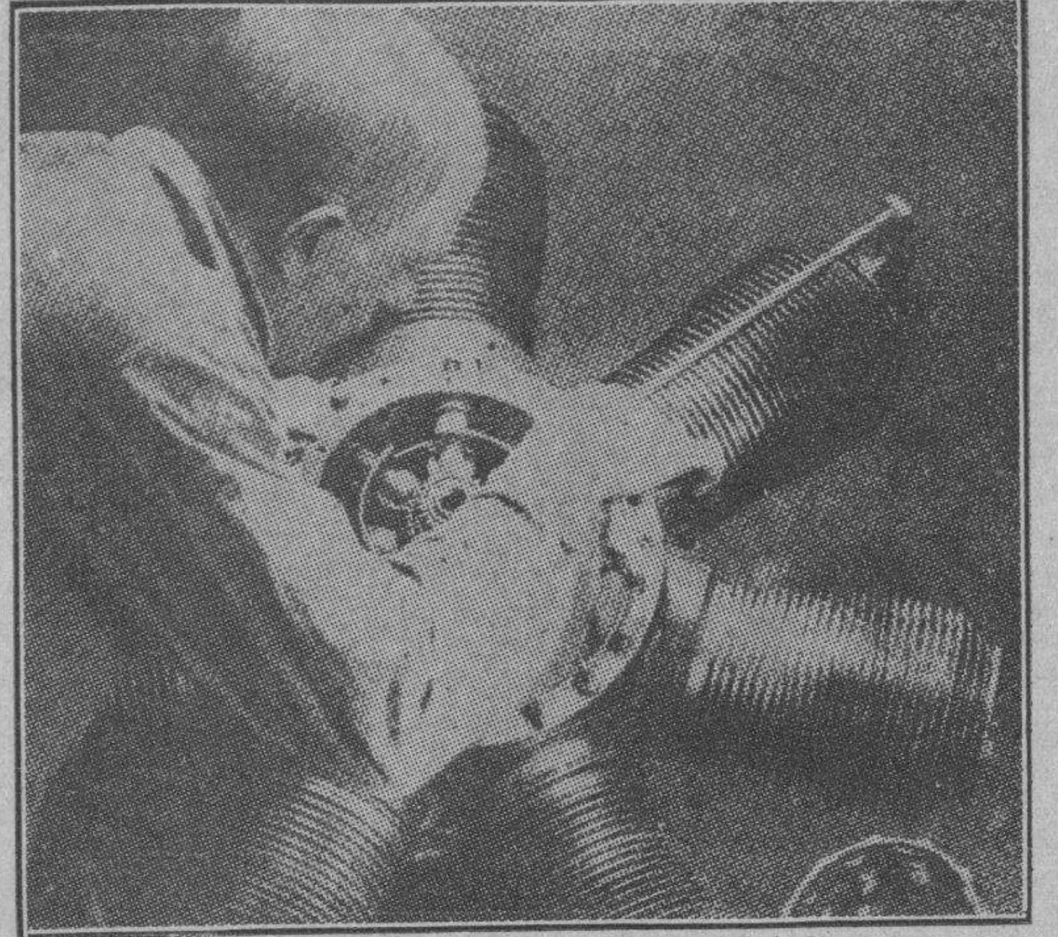
Un experto del Instituto de Ingenieros de Transporte, armando un motor radial, de aviación.
