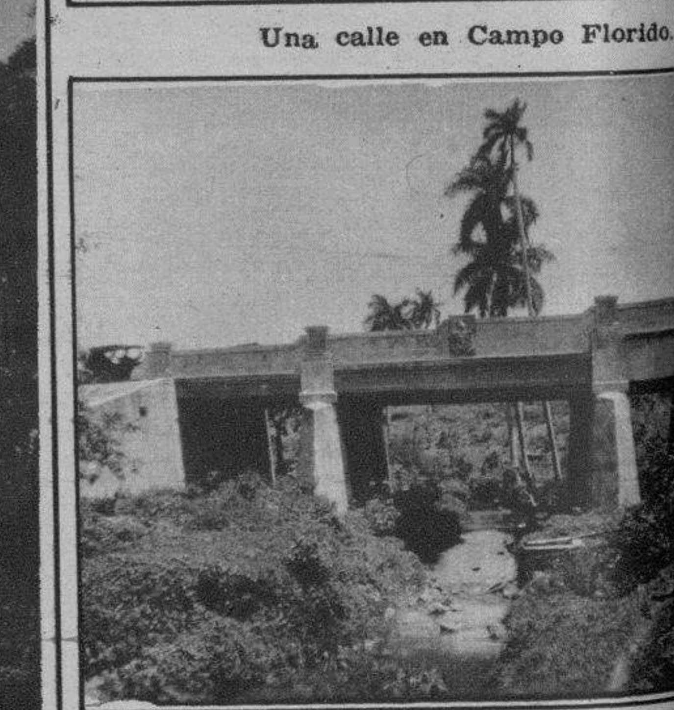
Puente en rampa sobre el río Quibús, en Madruga.
