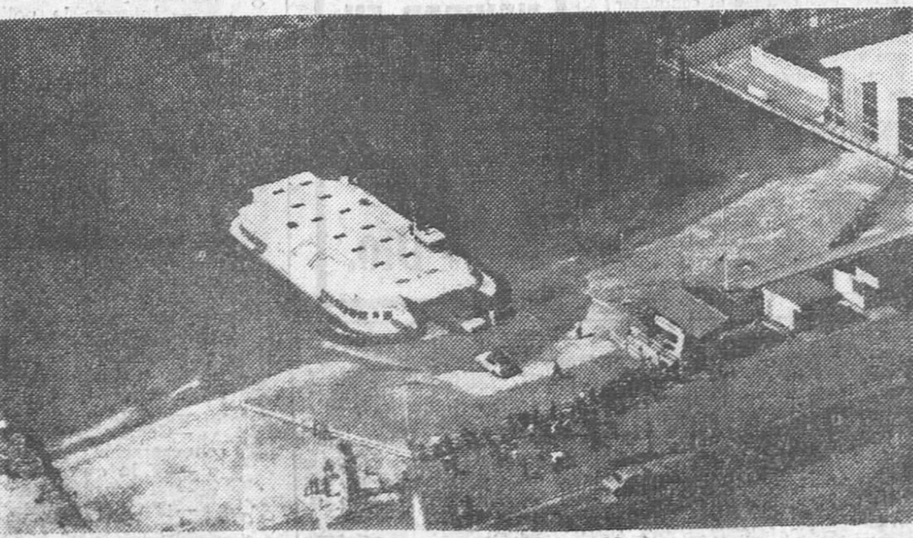
El prototipo VT-1 del Vospert Thornycroft, aparece en la ensenada de atraque de la costa Azul de Inglaterra, después de la realización con pleno éxito de las pruebas con una carga de hasta 102 toneladas. El VT-1 emplea hélices marinas sumergibles normales, en lugar de hélices aéreas. Dos turbinas de 1.000 caballos cada una proporcionan la potencia a los ventiladores que elevan la embarcación sobre un cojín de aire recubierto de caucho. El VT-1 puede asentarse sobre una playa. — (Foto FIEL)
