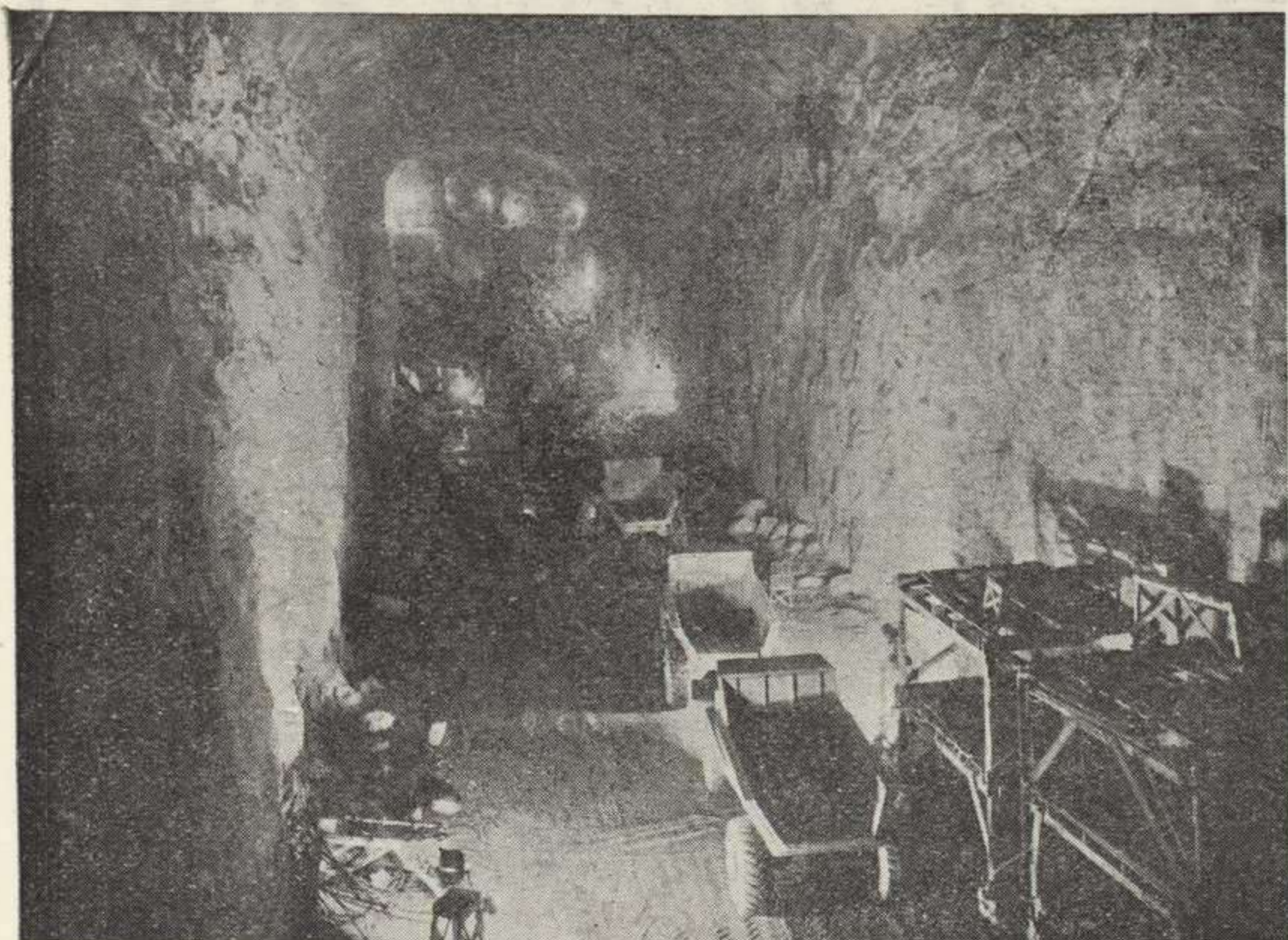
También en esta foto que nos muestra la destroza destinada a alojar el Cuerpo superior de la futura Central, se aprecian sus gigantescas dimensiones. En esta nave excavada en la roca se alojarán en su día los 6 grupos de que constará esta Central de Aldeadávila, con una potencia de 762.000 KVA y una producción anual de 1.700 millones de KWh. de energía regulada.
