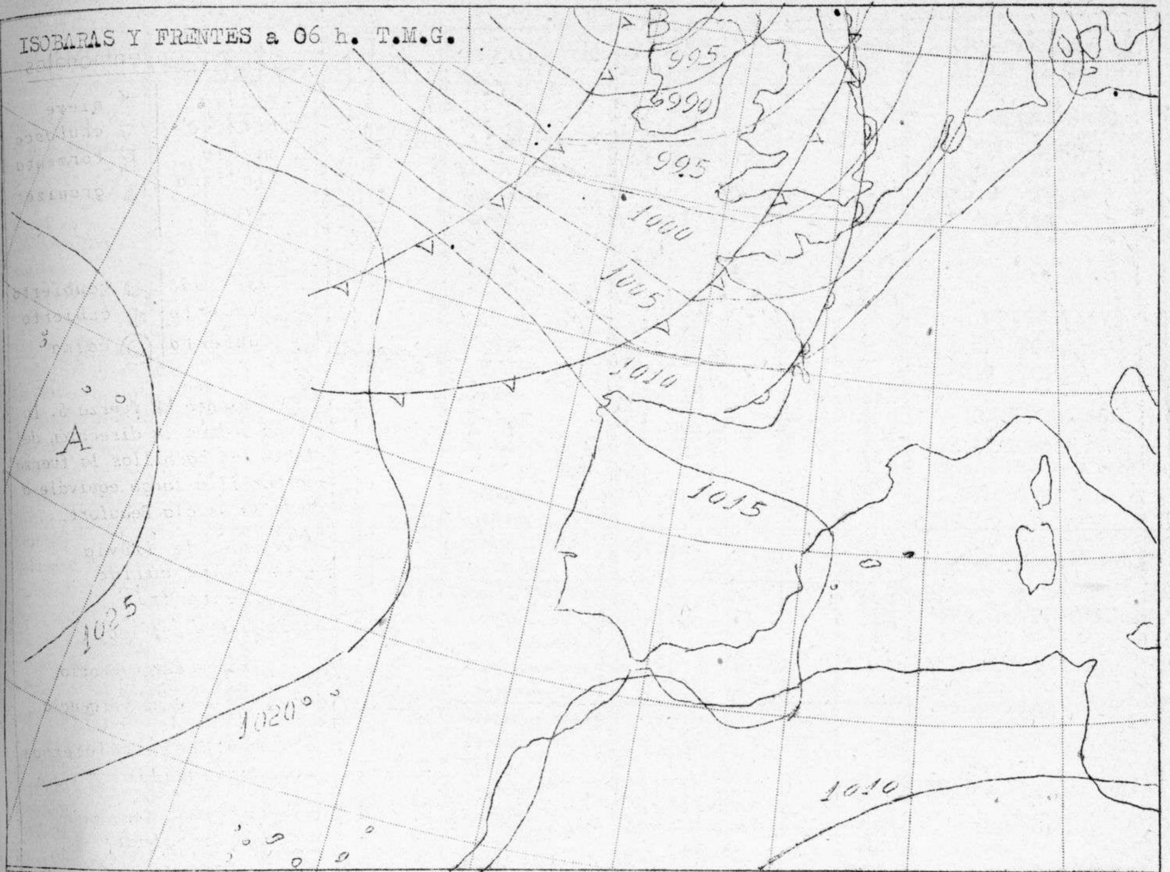
ISOBARAS Y FRENTE a 18 h. T. M. G.
