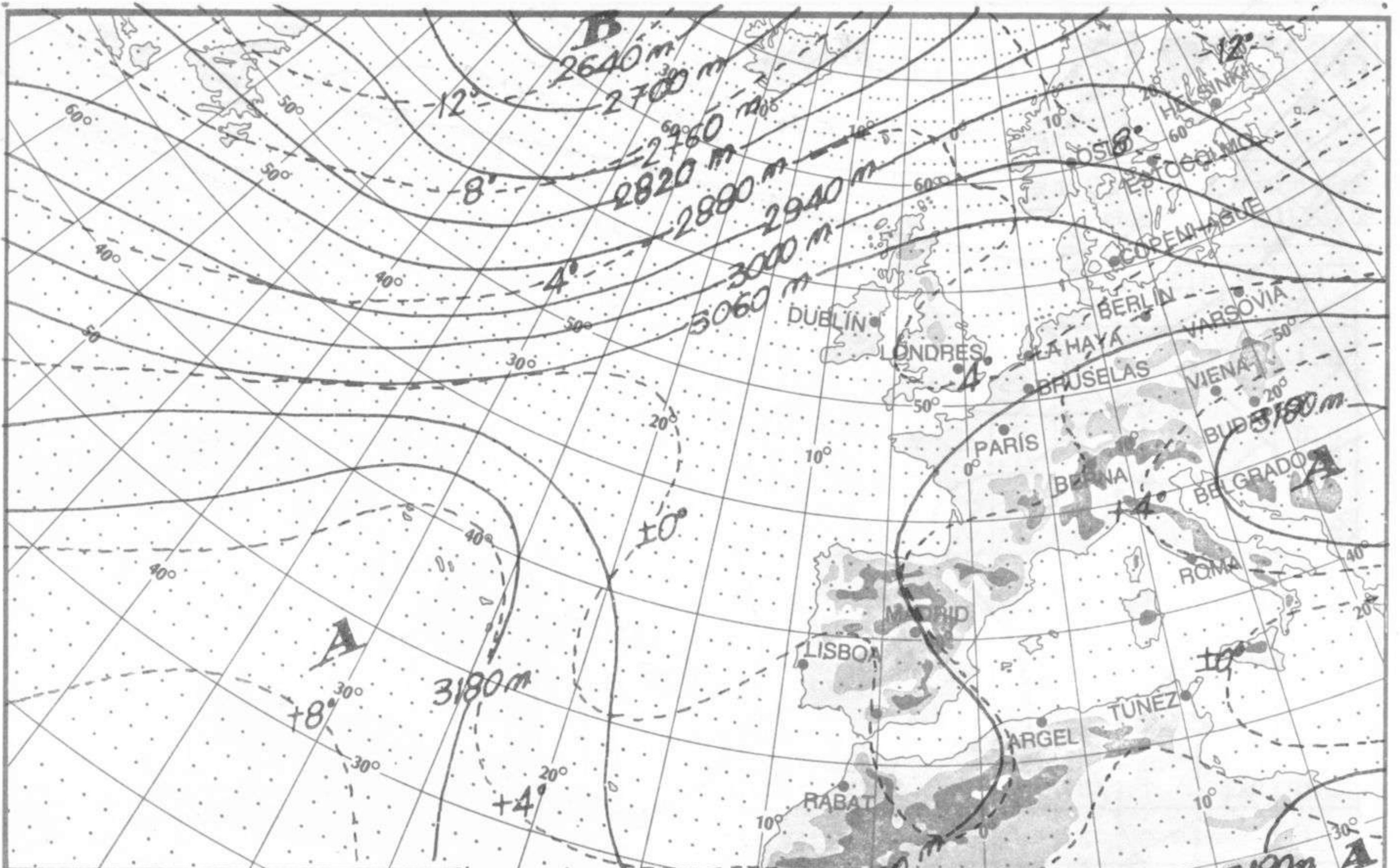
TOPOGRAFIA DE LA SUPERFICIE DE 700 HPa a 12 h. (TMG) Día 11-10 -86
