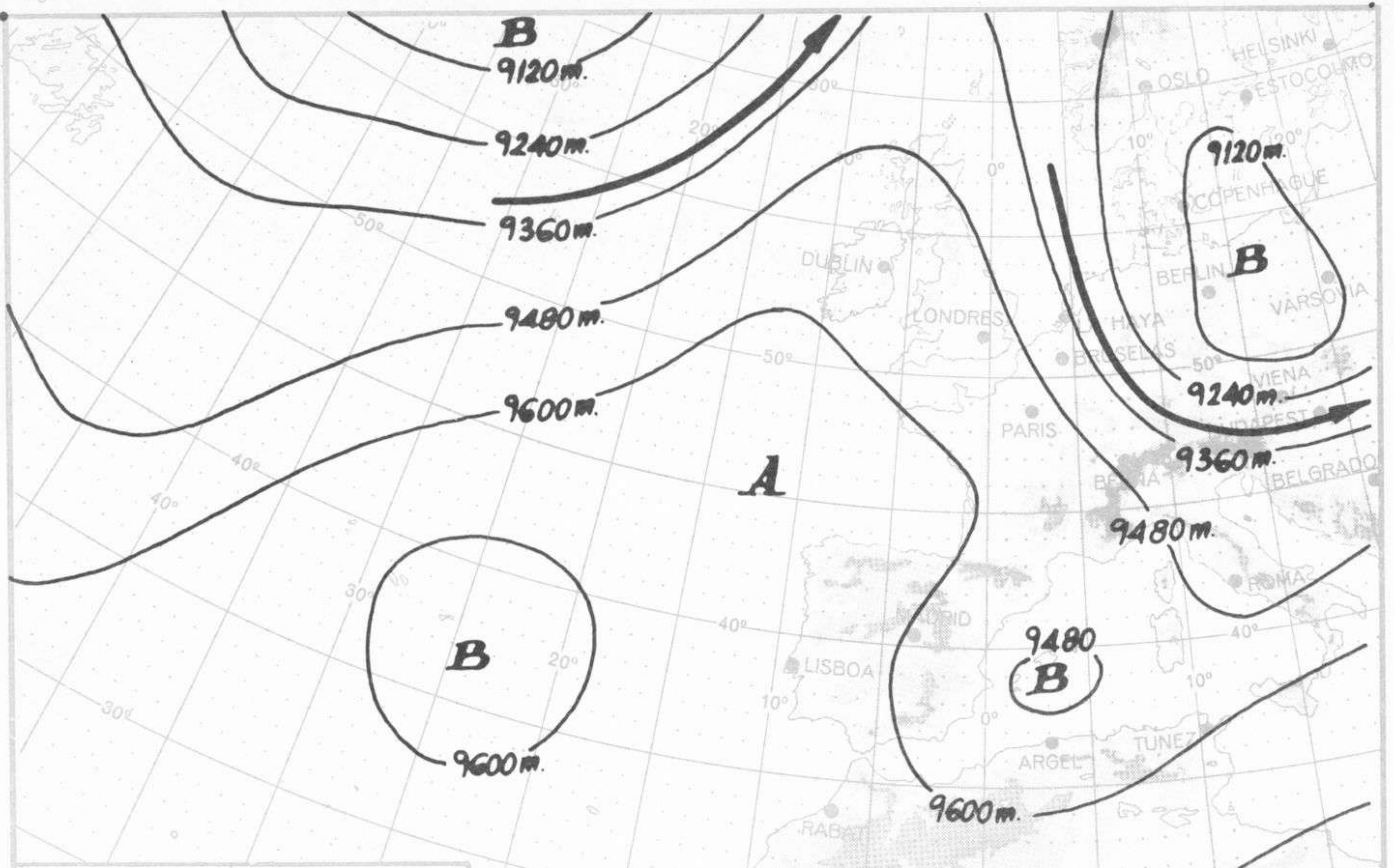
TOPOGRAFIA DE LA SUPERFICIE DE 300 mb. a 12 h. (TMG) Día 23-8-81.
