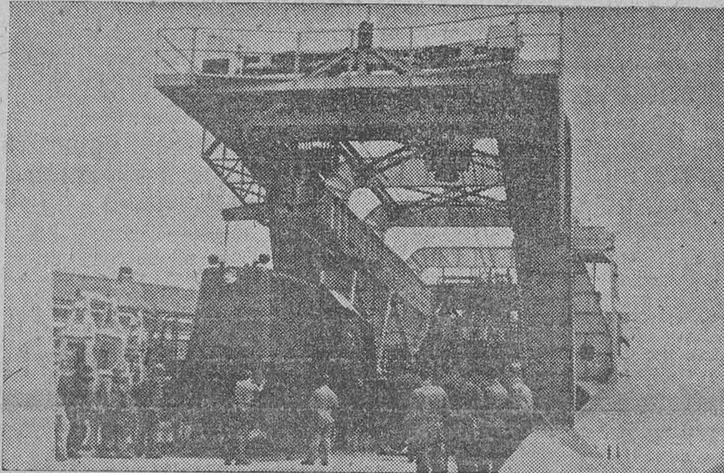
Otra de las grandes innovaciones aliadas que ayudó a ganar la guerra, fué el buque transporta-trenes, construido por ingenieros británicos. En esta (foto) vemos a uno de estos buques admitiendo a un tren eléctrico completo, que fué transportado desde Inglaterra a Francia, y que comienzan a funcionar en el mismo momento en que entran en los railes. — (Foto Logos.)
