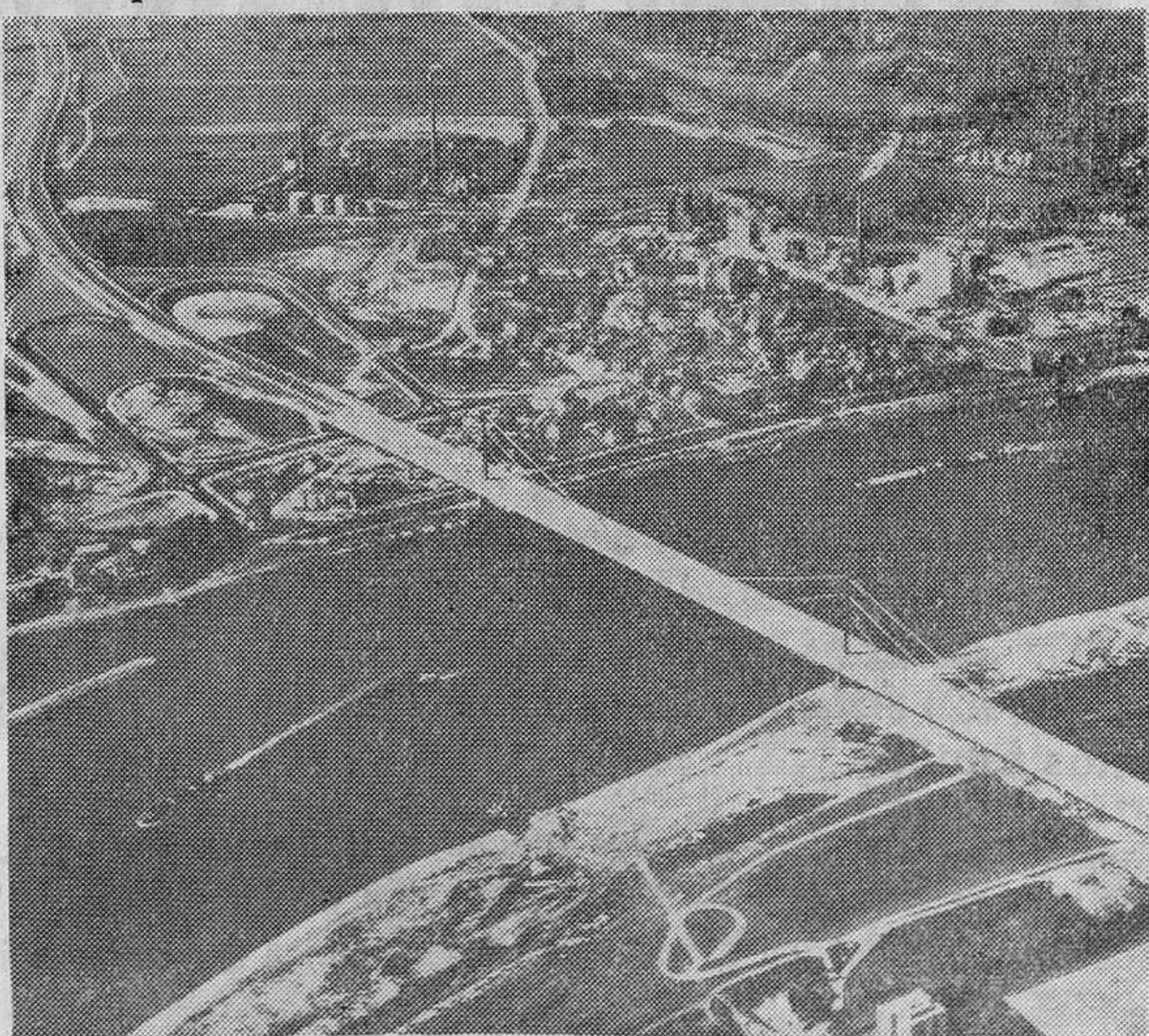
El nuevo puente sobre el Rhin, cerca de Duisburg, constituye el mayor puente de acero del mundo, de cables oblicuos, de vigas centrales, de construcción soldada, sin remaches algunos. Sus características técnicas: 778 m. de largo, 350 m. de luz, 36,3 m. de ancho, con seis calzadas, pistas para ciclistas y veredas para peatones. Invertiéronse diez mil toneladas de acero en la obra. De los 25 puentes nuevos sobre el Rhin (hoy existen 34), proyectados por Bonn hasta fines de los años ochenta, cinco se encuentran ya en vías de ejecución
