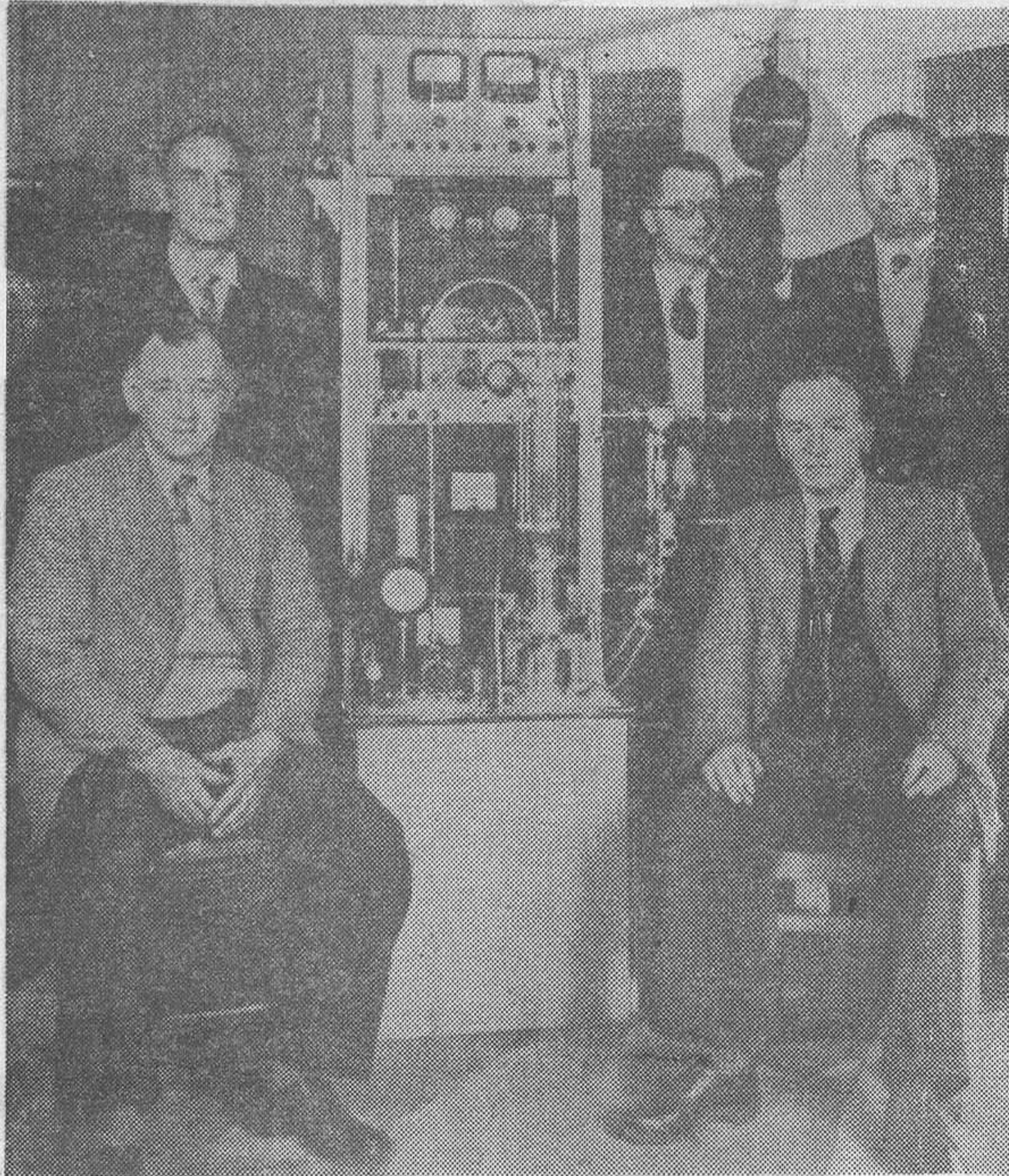
Para medir el tiempo con la exactitud exigida por la técnica y la investigación modernas, se emplean muchos y variados procedimientos. Este, que muestra la foto funciona a base de moléculas de gas amónico que vibran produciendo 24.000 millones de impulsos eléctricos cada segundo. Construido en Inglaterra para servicio postal australiano, se calcula que sólo variará un segundo en veinticinco años.
