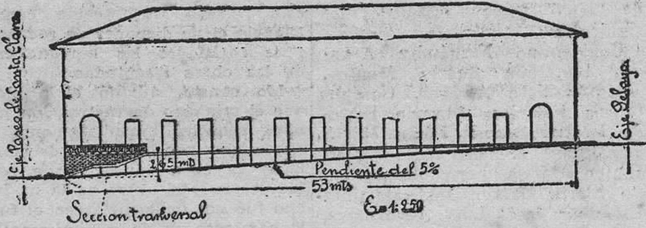
Fachada oeste del Teatro Campoamor y sección transversal de la rampa que podría sustituir a la escalinata, con una pendiente del cinco por ciento.
