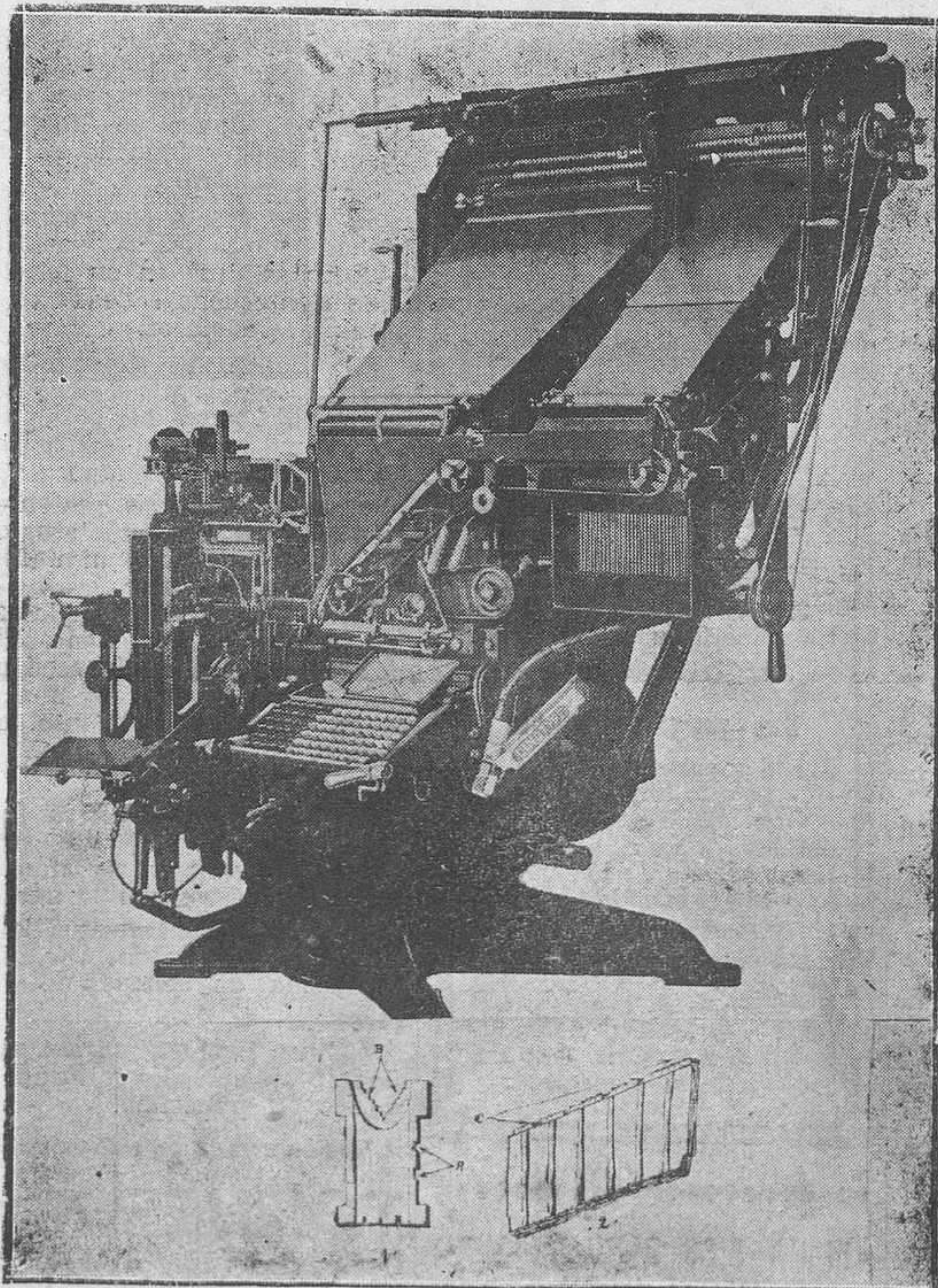
1.-Matriz de la "Linotipia".—A. Dientes para la distribución de las matrices en la Linotipia.—B. Lugar en que se hallan grabadas las letras.—C. Línea hecha y fundida.—2.-Línea hecha y fundida.—C. Lugar de las letras.
