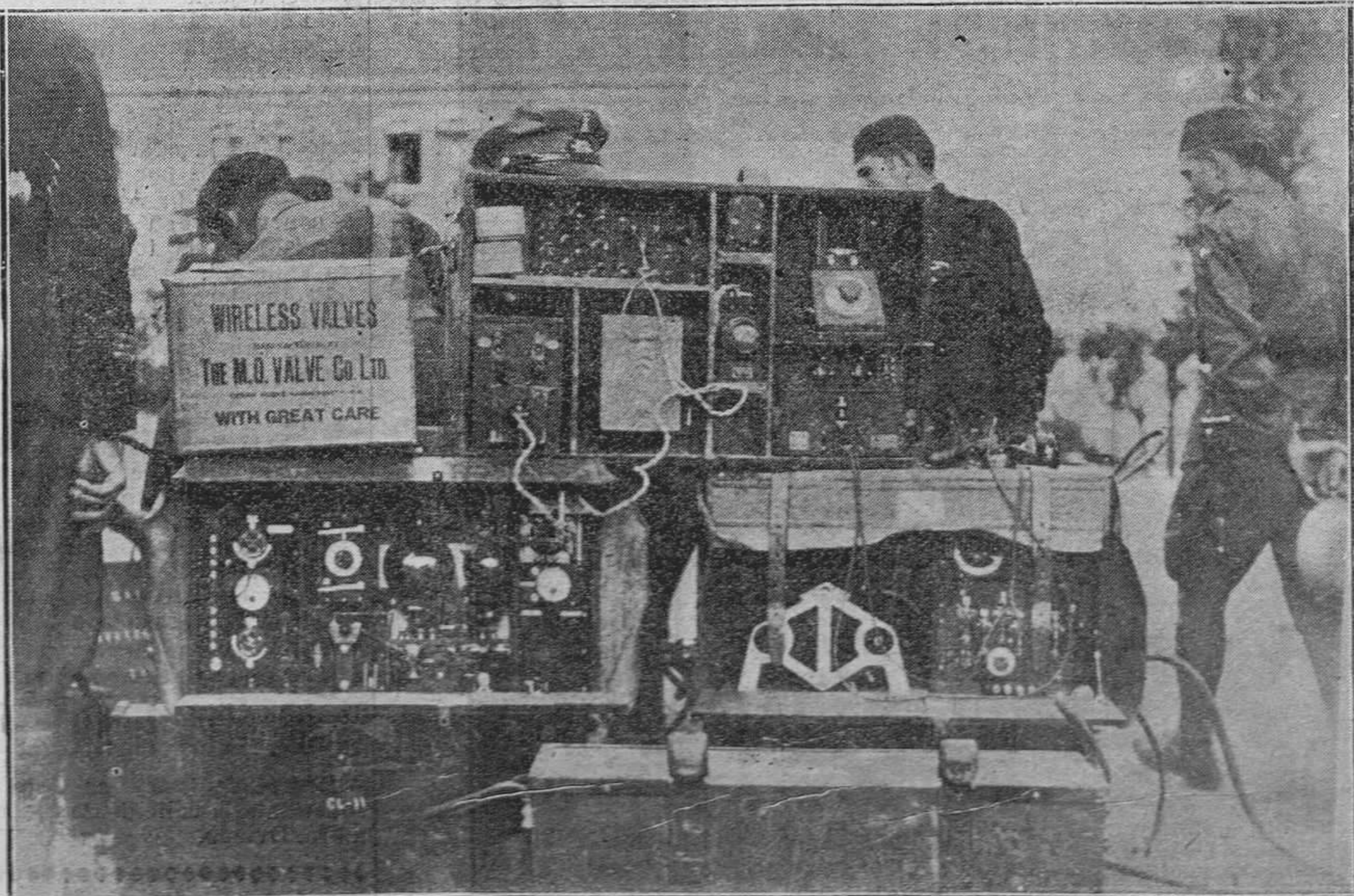
OVIEDO.-La estación radiotelegráfica de la compañía de la Escuela práctica del Centro Electrotécnico, que anteriormente estuvo en esta ciudad. (Foto Buelta)
