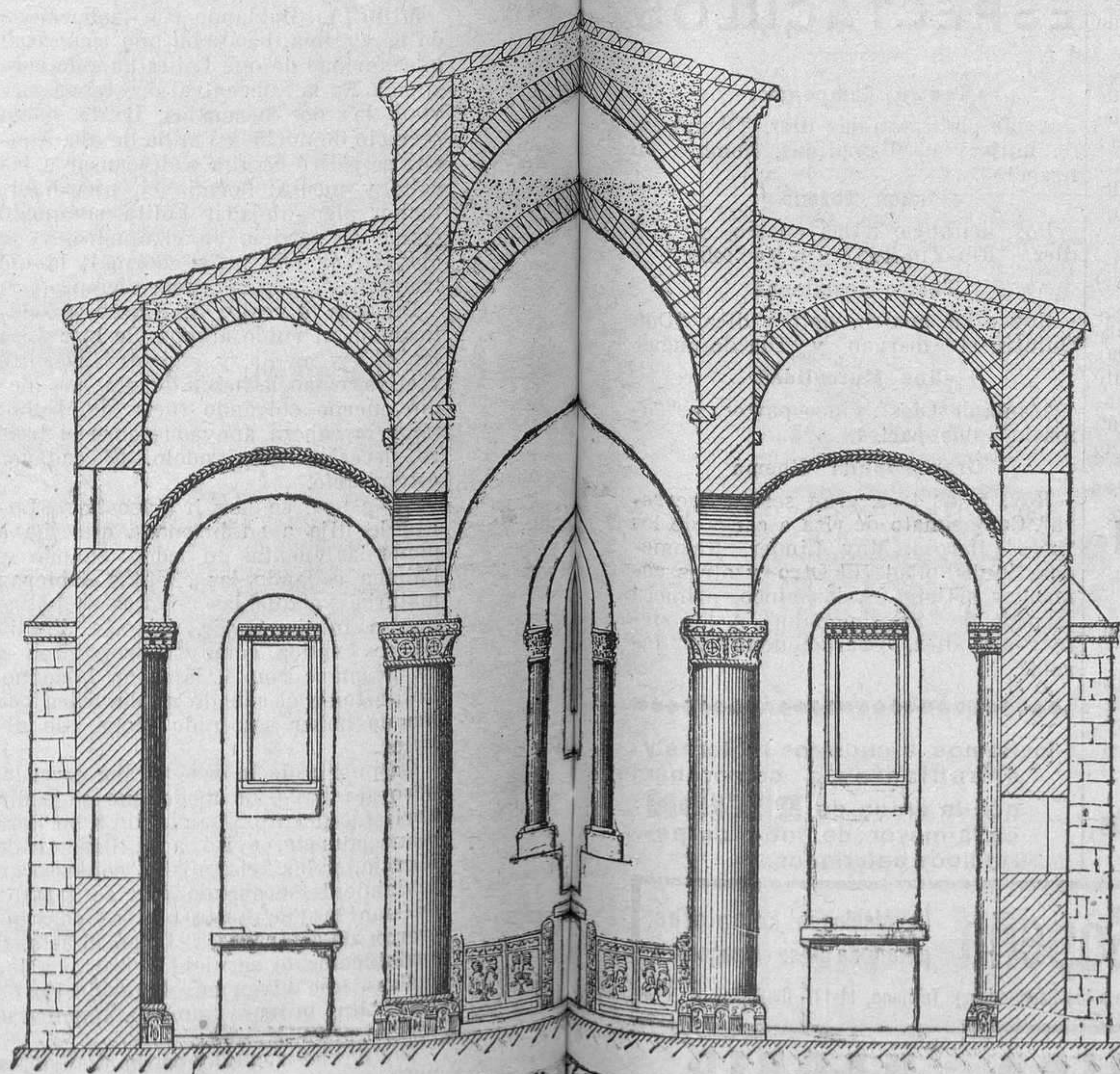
Fig. 9.-sección longitudinal por el eje de la figura 5.
