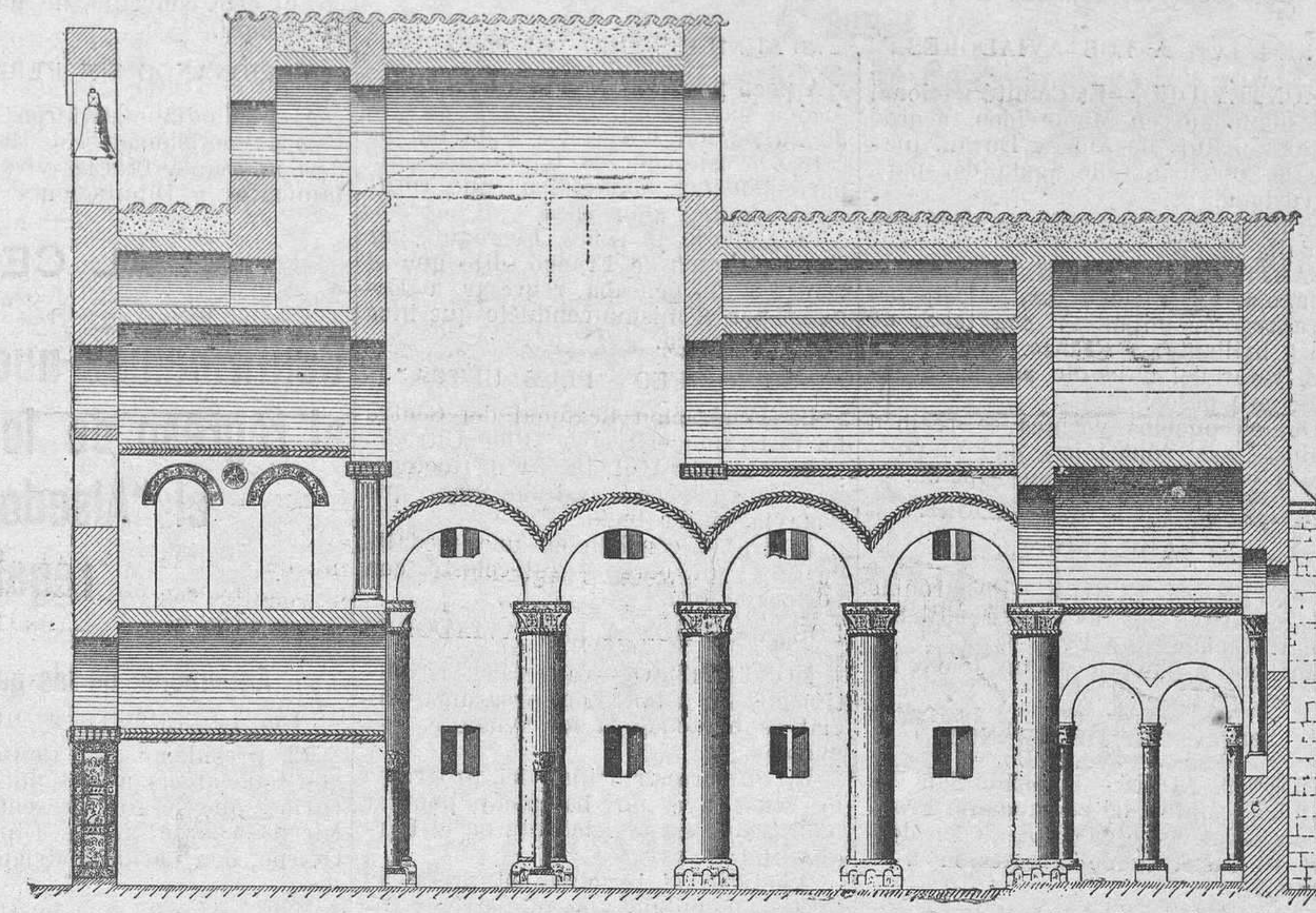
Fig. 8.-Sección conjitunal por el eje de la figura 5.
