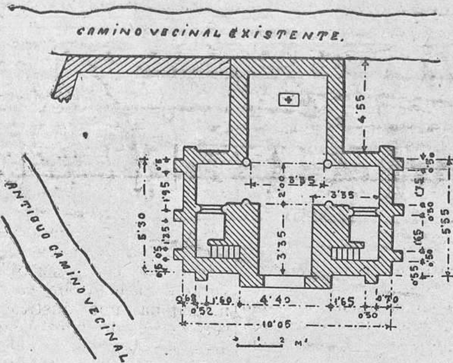
Fig. 2.-Planta que hoy ocupa el templo de San Miguel de Lillo.
