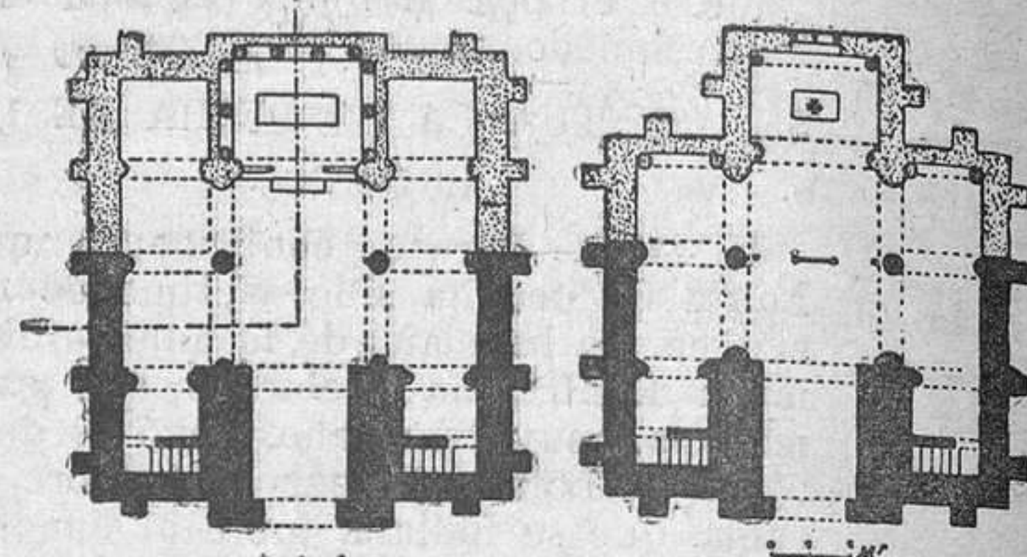
Fig. 6.-Planta restaurada por el señor Lampérez
