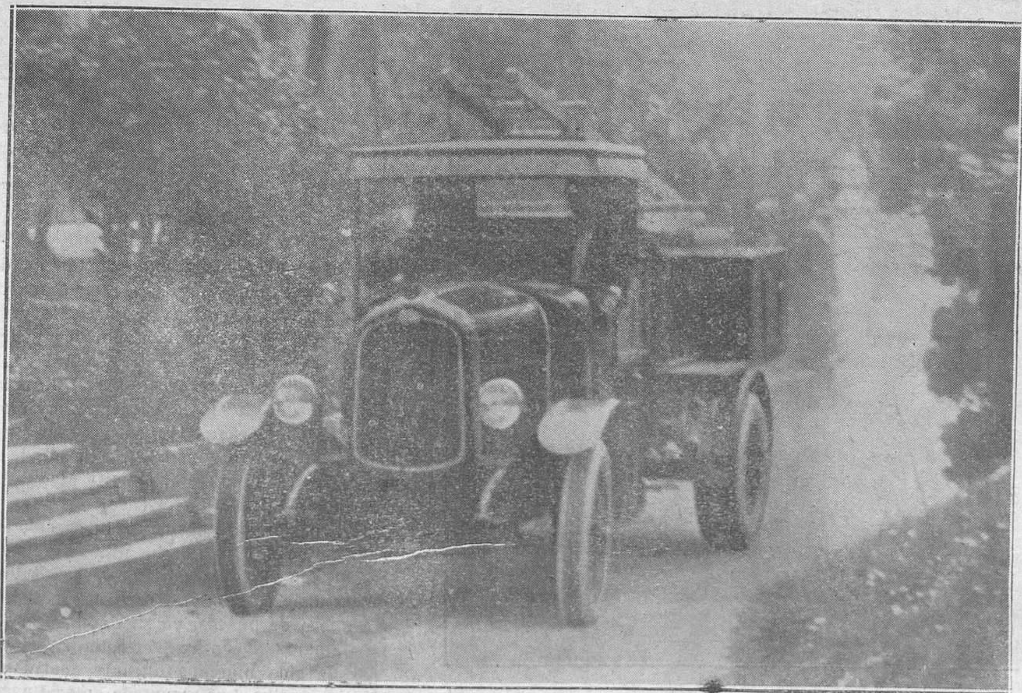
La autobomba automóvil para el servicio de riego e incendios, cuyas pruebas fueron efectuadas ayer en el Bombé. (Foto Buelta)
