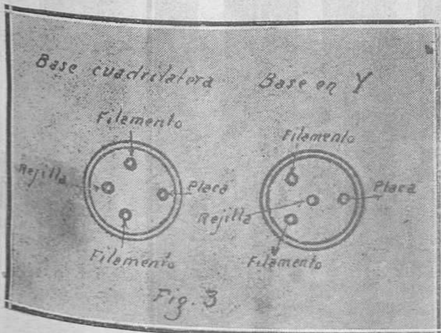
Fig. 3.--Disposición de los enchufes.
