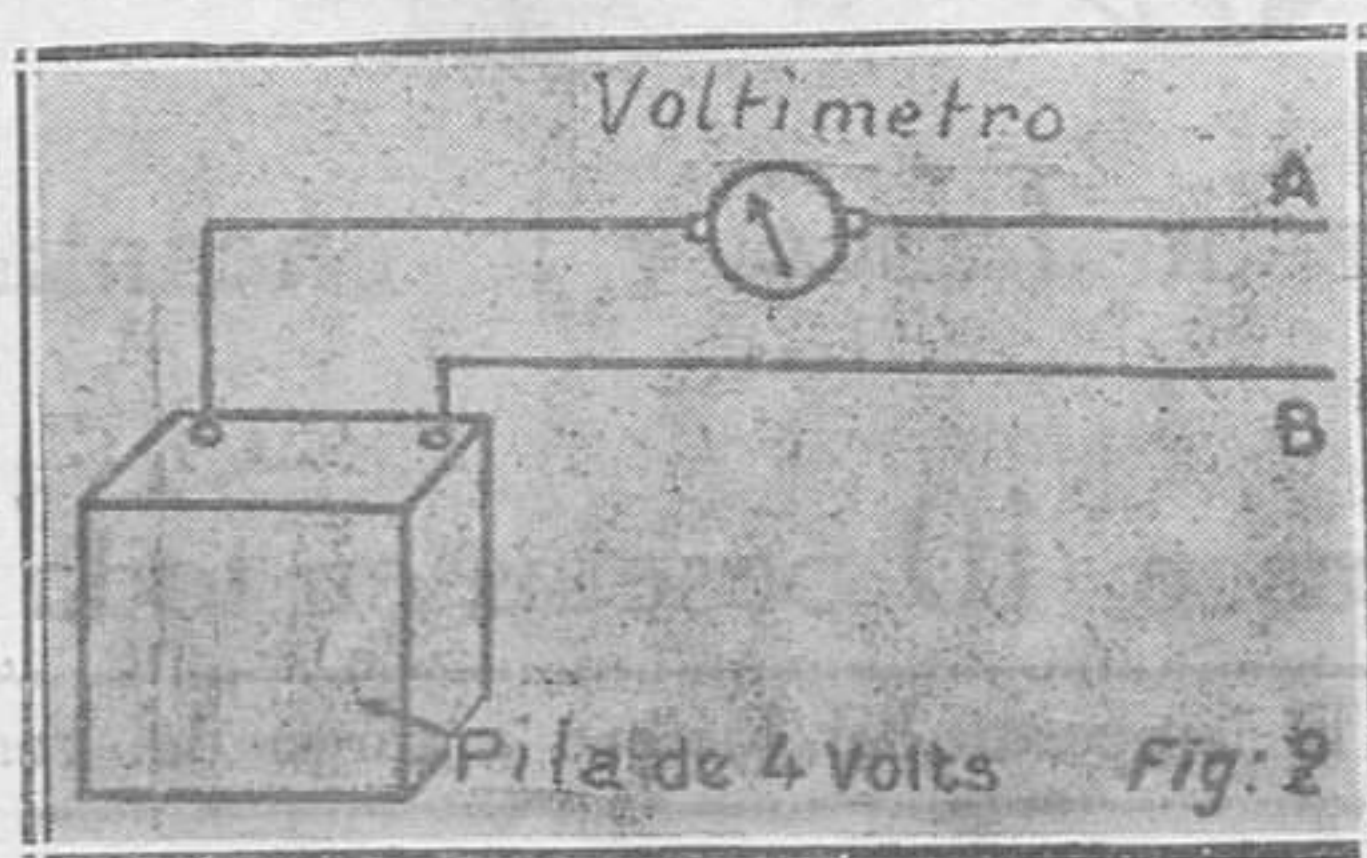
Fig. 2.--Modo de averiguar si el filamento de la lámpara se halla en buenas condiciones.
