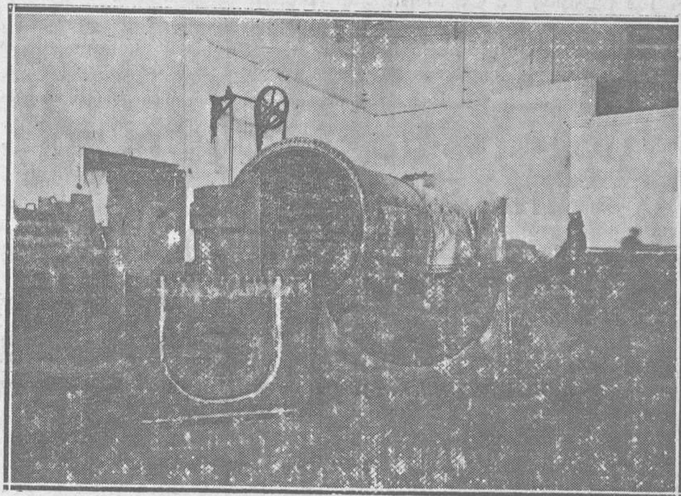
La capacidad de los grandes talleres. con sus obreros especializados y elementos técnicos directivos, tienen en este grabado una nueva muestra al prepararse otra caldera de locomotora para la soldadura autógena y eléctrica, el moderno procedimiento de reparación.
