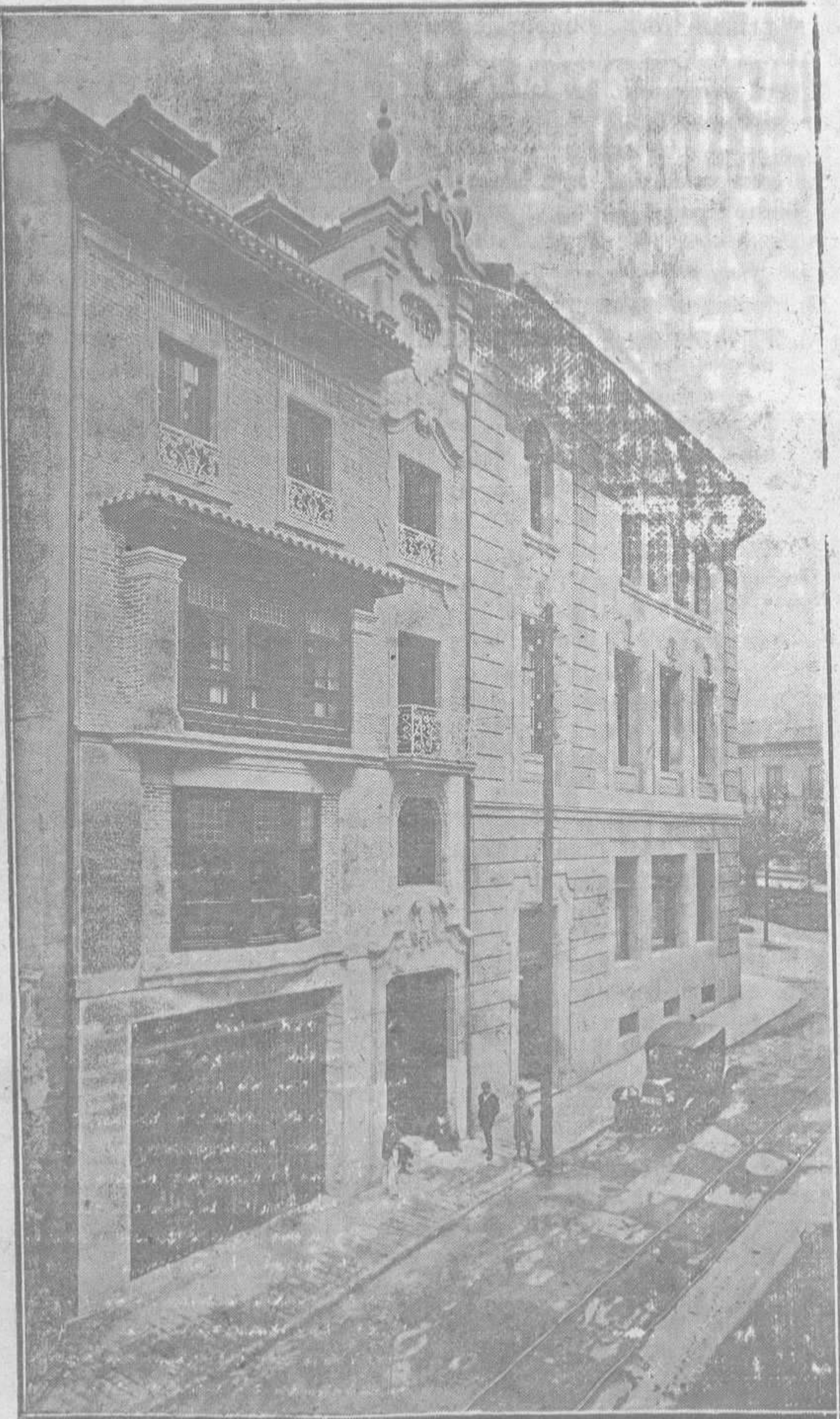
Un trozo del Oviedo moderno, en la calle de Mendizábal, donde se destaca por su elegancia y carácter la casa cuya construcción acusa la personalidad del arquitecto señor Bustelo.
