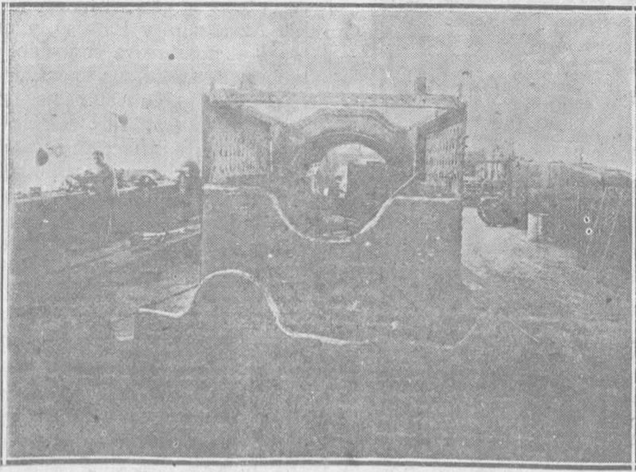
Calderas de una máquina de mercancías del Ferrocarril Vasco, preparadas para la aplicación de la soldadura autógena y eléctrica, siendo éste el primer Ferrocarril de Asturias que empleó dicho procedimiento en sus Talleres.
