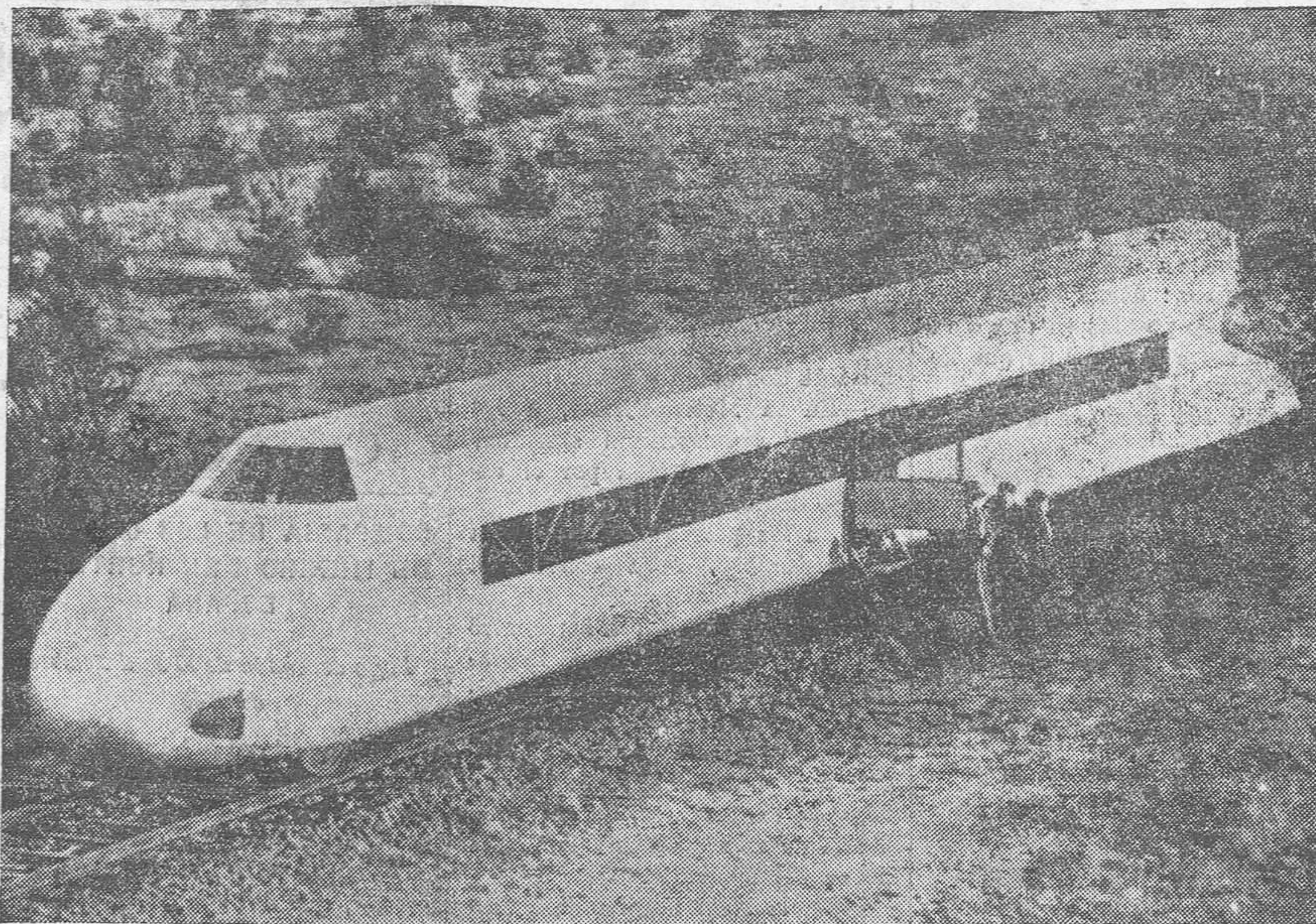
Curiosa fotografía del «tren del porvenir». Bólide construido por el ingeniero H. Kruekeburg, en Hannover, que desarrolla una velocidad de 160 kilómetros por hora, movido por motor de aviación de 200 H. P. y hélice, siendo su peso de 18.500 Kilos, 26 metros de largo y cabida para 40 pasajeros.
