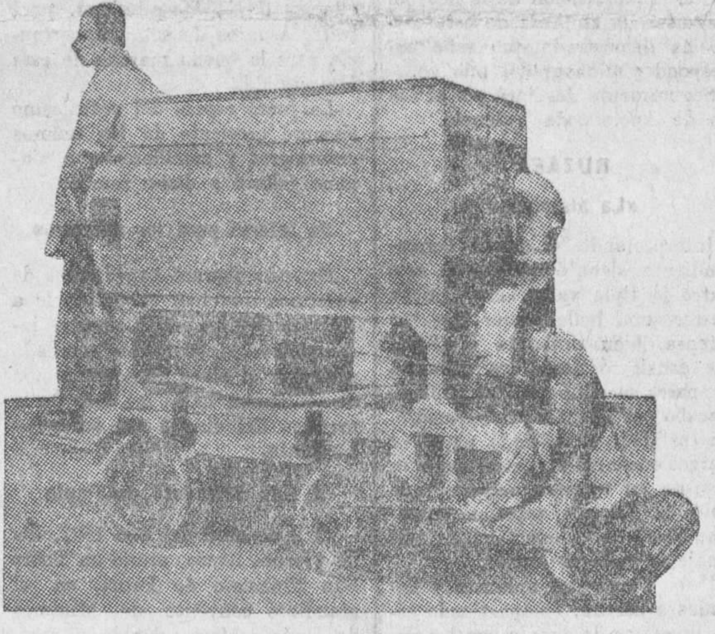
La nueva máquina barredora que está funcionando en Nueva York
