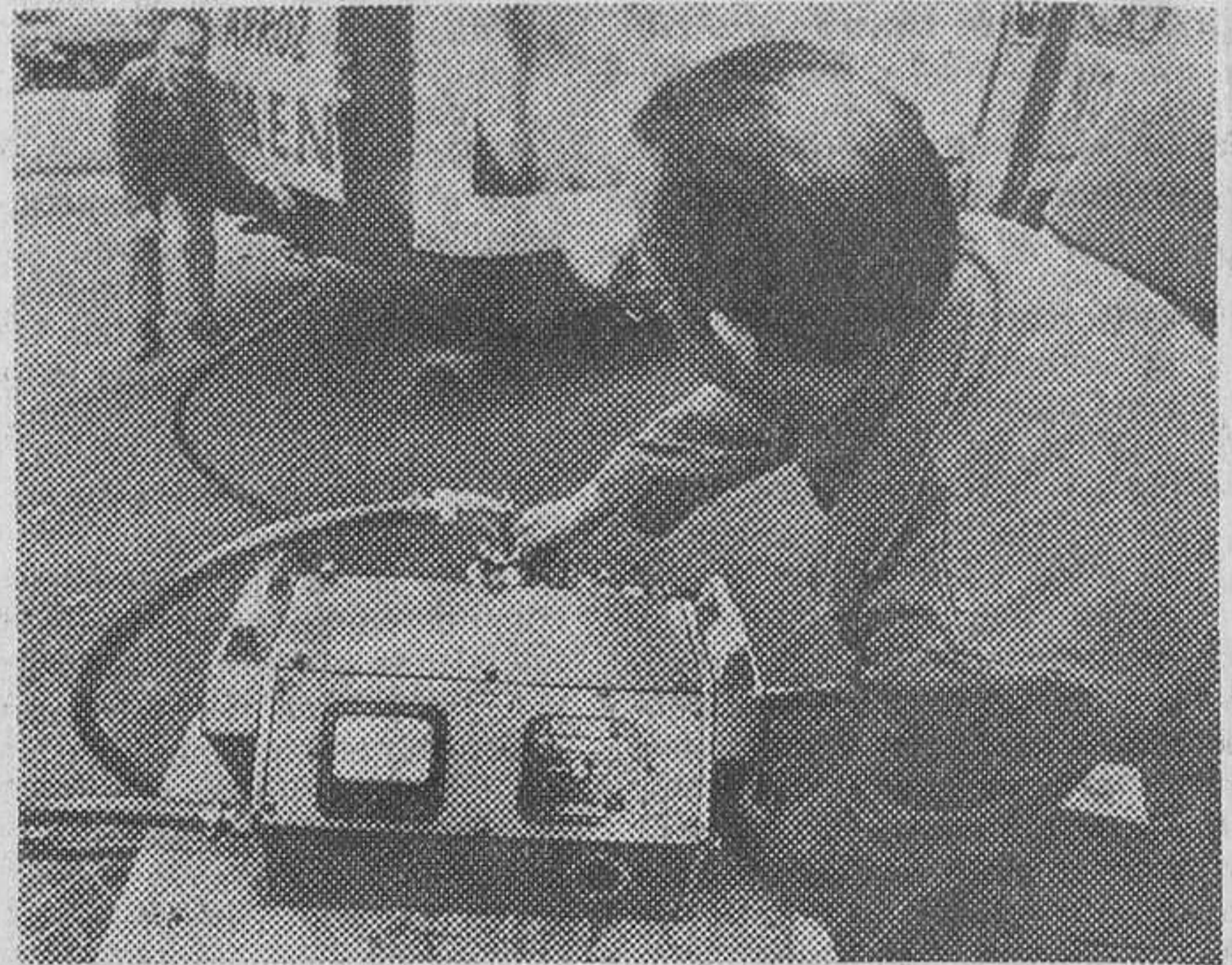
Este es el aparato medidor de humos utilizado para controlar los autobuses de Barcelona. (Foto Soterias.)
