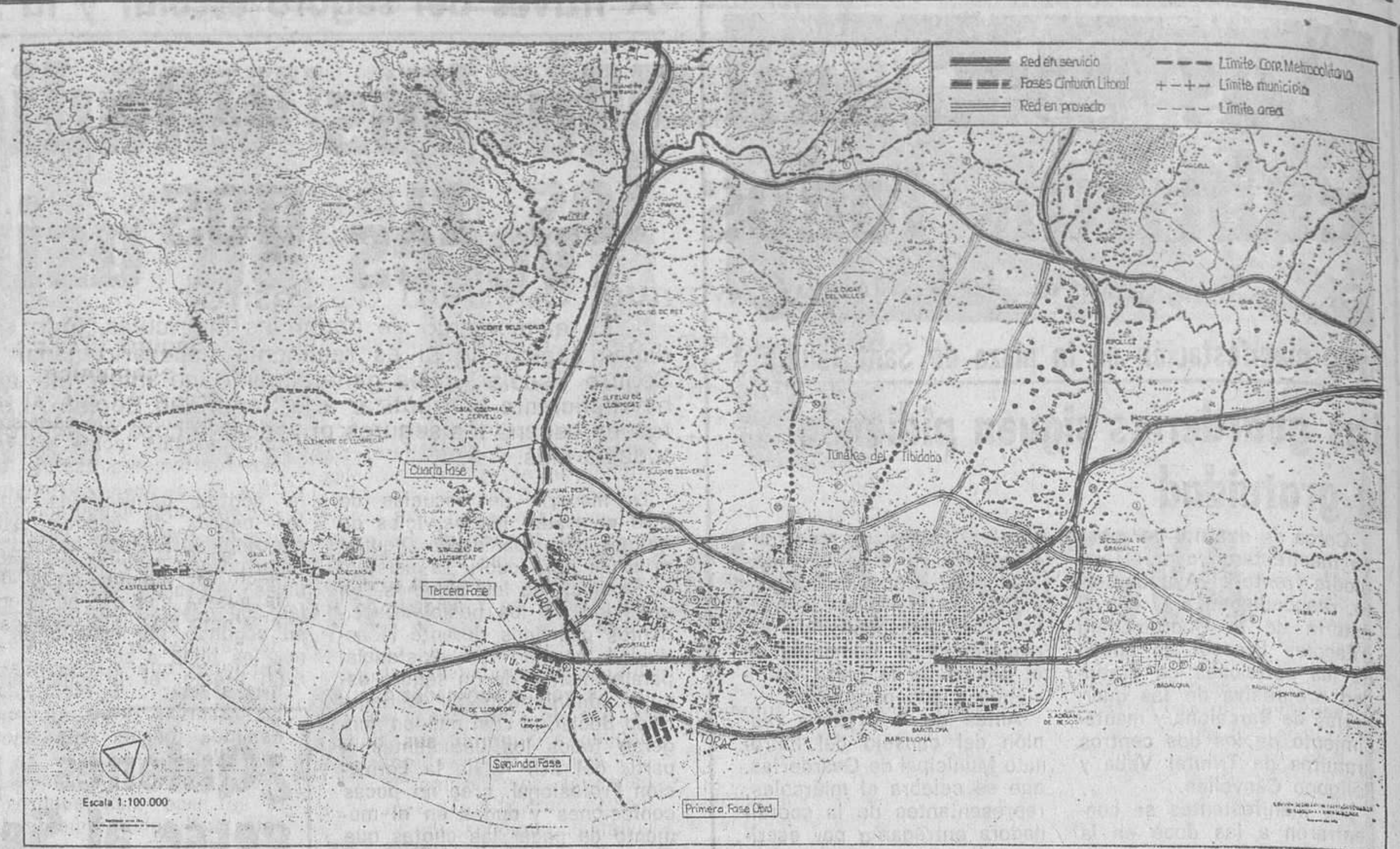
Plano esquemático de la red viaria barcelonesa. A la izquierda aparece el Cinturón del Litoral, que permitirá enlazar el Puerto y la Zona Franca con la autopista de Molins de Rei. El Cinturón atravesará el Puerto mediante un túnel o un puente —representado mediante puntos continuos— para dirigirse hacia las autopistas del Maresme y el Vallès
