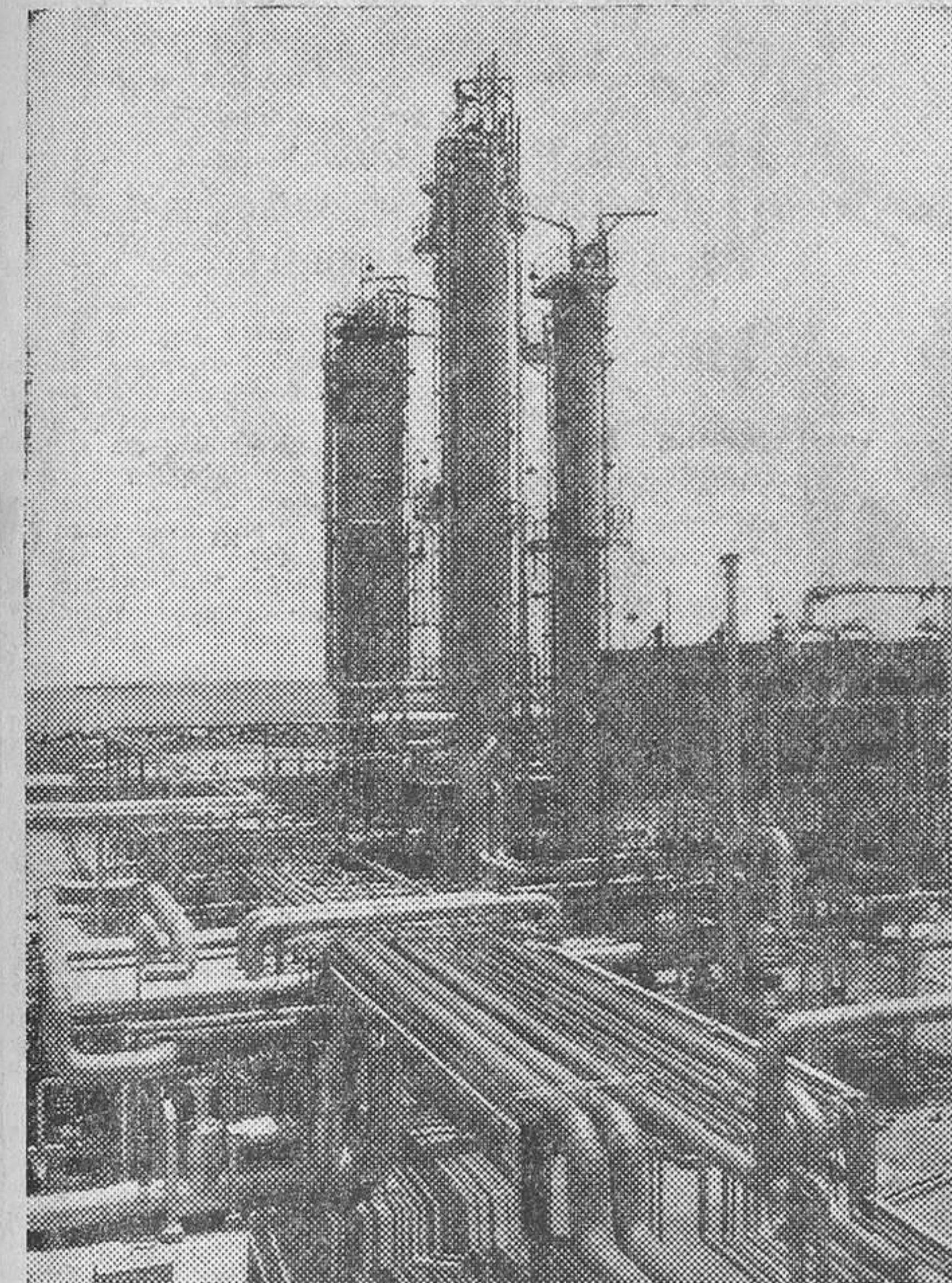
La terminal de Barcelona fue la primera del mundo en la que se practicó el fraccionamiento del gas natural libio en sus distintos componentes: metano, etano, propano, butano y naftas
