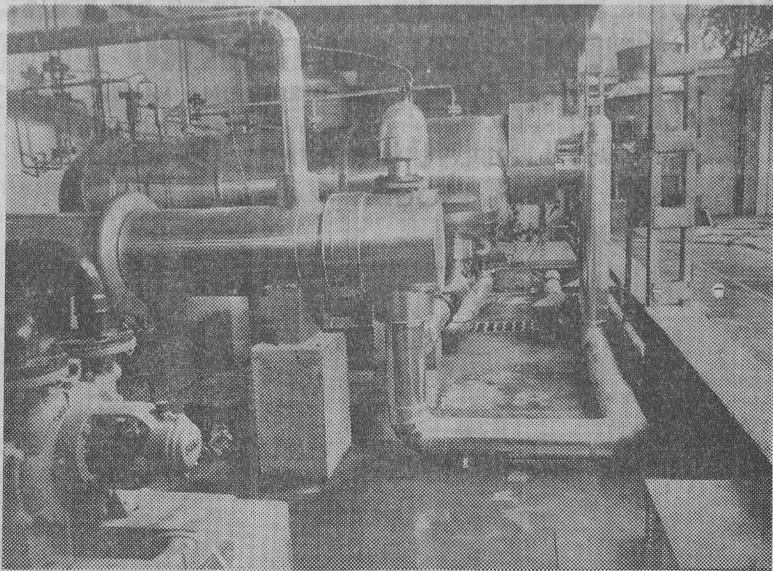
Planta piloto de desalación de agua de mar, instalada en terrenos de la Junta de Energía Nuclear, en Madrid. — (Foto Europa Press.)
