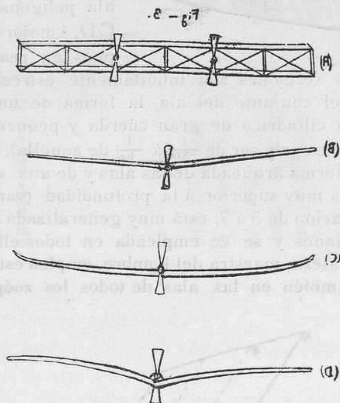
Fig. 3.—Perfiles longitudinales de un ala: (A) vértice, (B) en V, (C) perfil propuesto por Tatin, (D) ídem por el infrascrito
