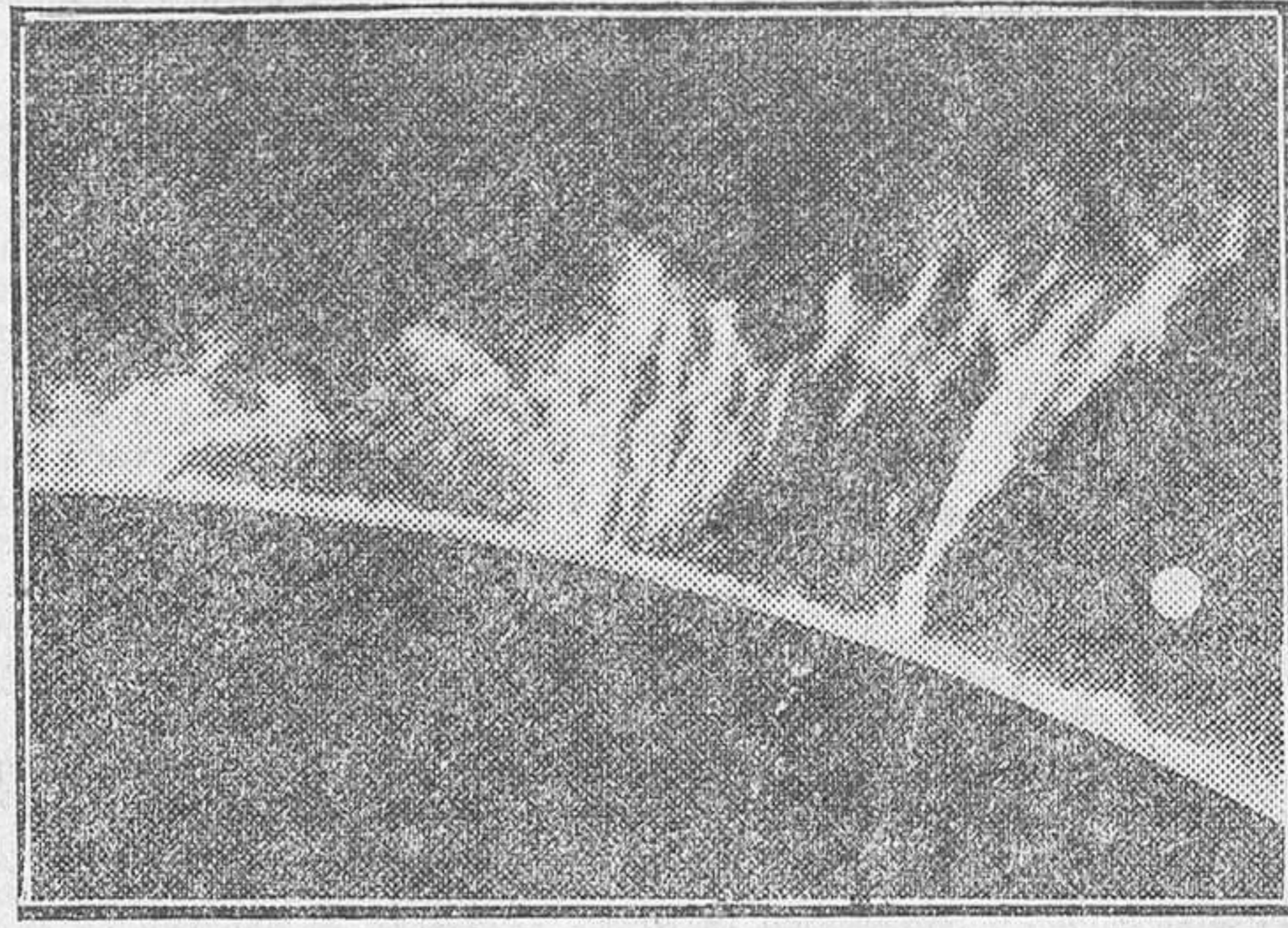
Protuberancias solares que alcanzan más de noventa mil kilómetros de altura, fotografiadas en el Observatorio de Monte Wilson. (El disco blanco simboliza nuestro planeta a la misma escala.)
