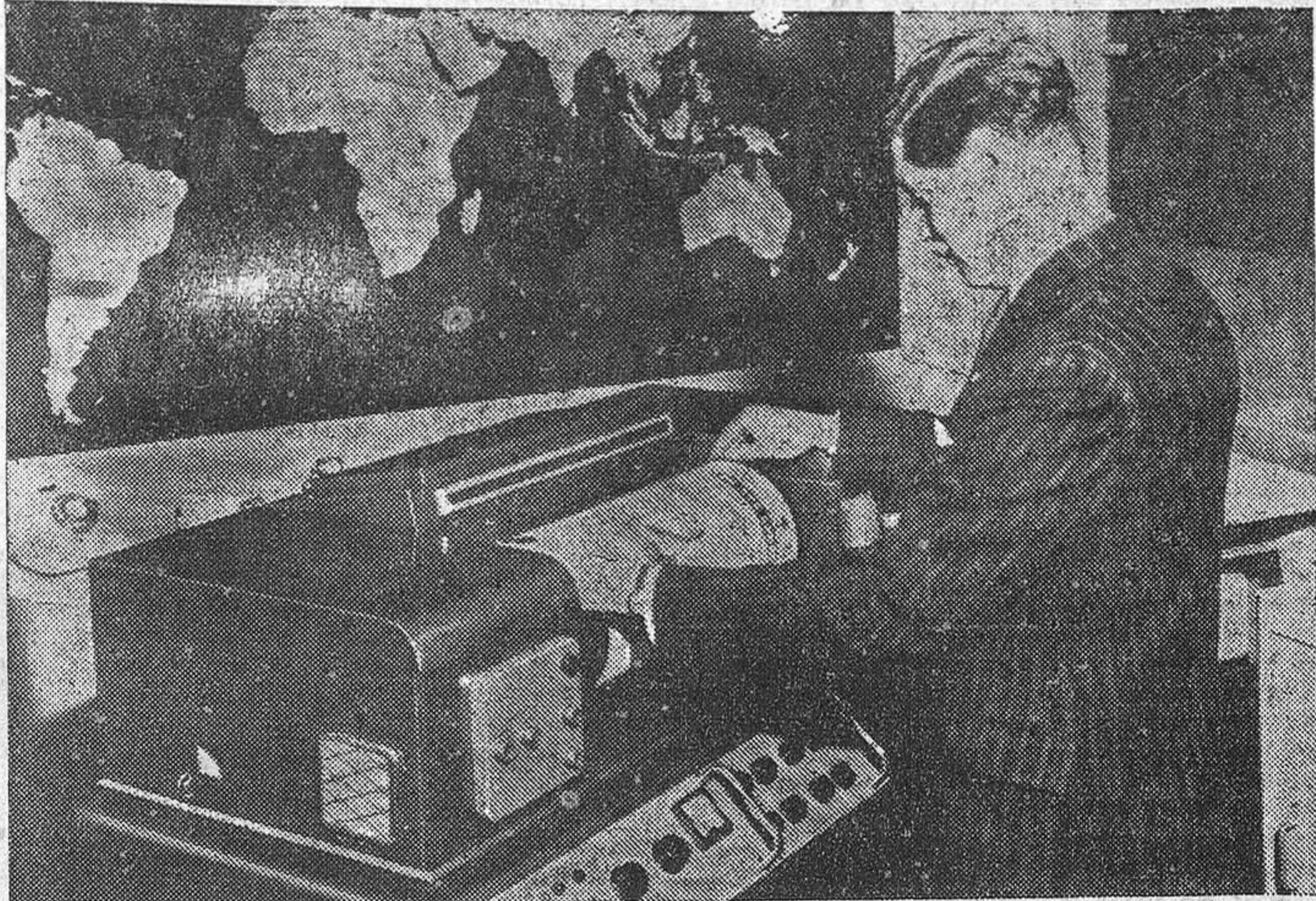
Un operador carga el cilindro del transmisor de páginas Muirhead por sistema facsimil, aparato que permite recibir copias fotográficas de originales a muchos centenares de kilómetros de distancia.
